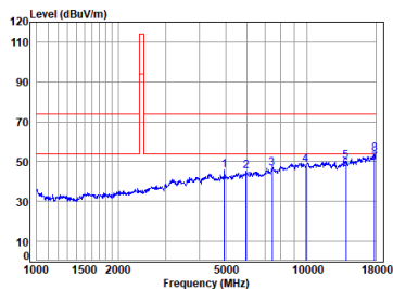
2.4G SRD_TX_CH_H_Horizontal
