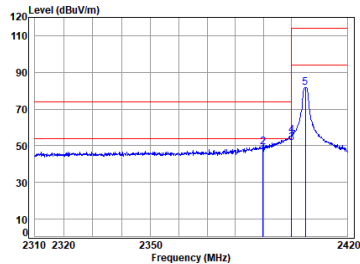
2.4G SRD_TX_CH_L_Horizontal
