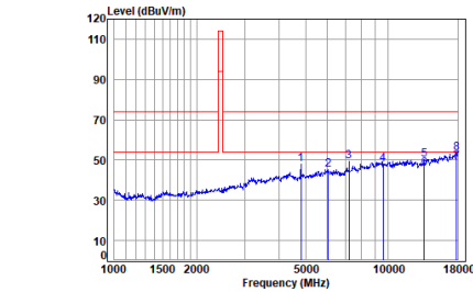
2.4G SRD_TX_CH_L_Horizontal
