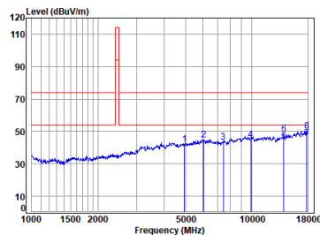
2.4G SRD_TX_CH_H_Vertical
