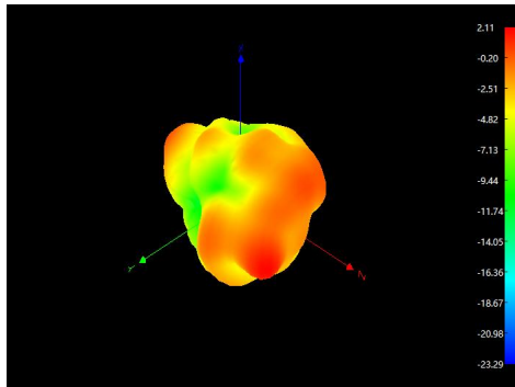
3D 2450MHz
