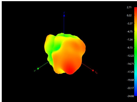
3D 2500MHz
