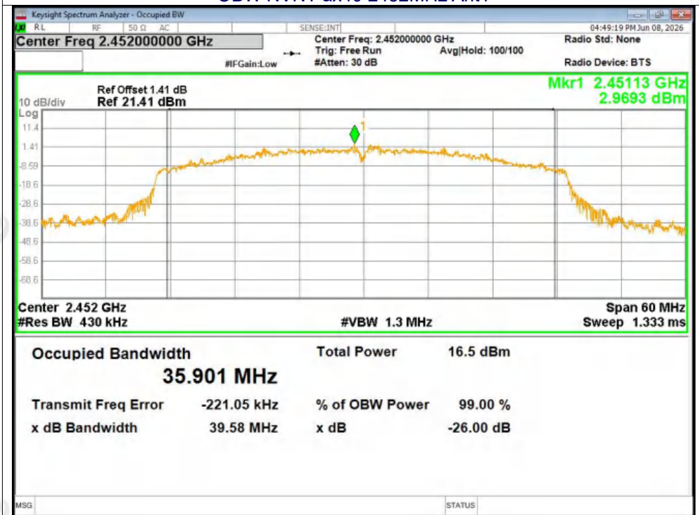
OBW NVNT ax40 2452MHz Ant1
