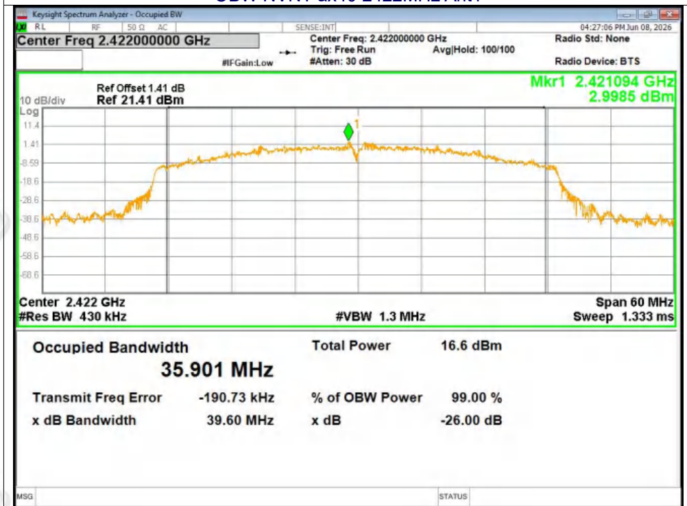
OBW NVNT ax40 2422MHz Ant1
