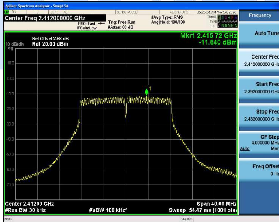
PSD g 2412MHz
