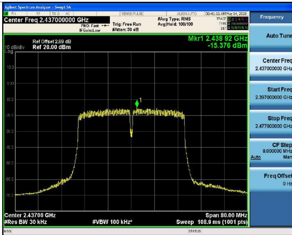
PSD n40 2437MHz
