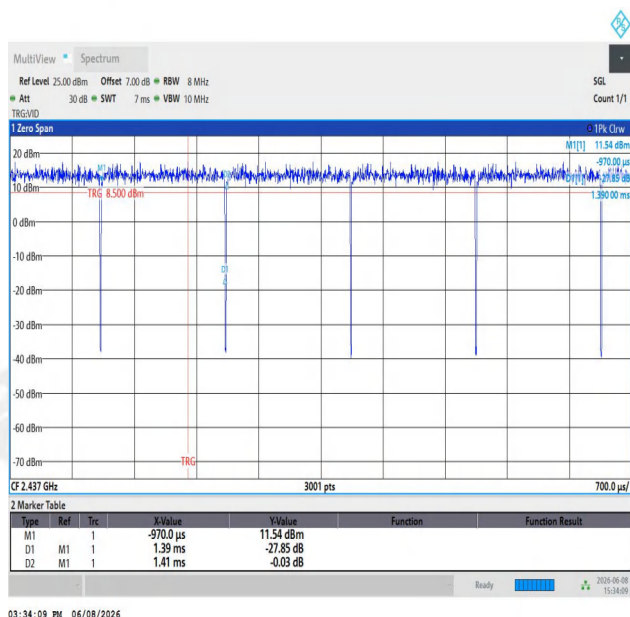
NTNV-11G-Ant1-2437
