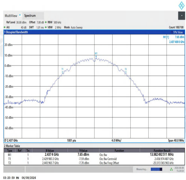
11B-Ant1-2437
