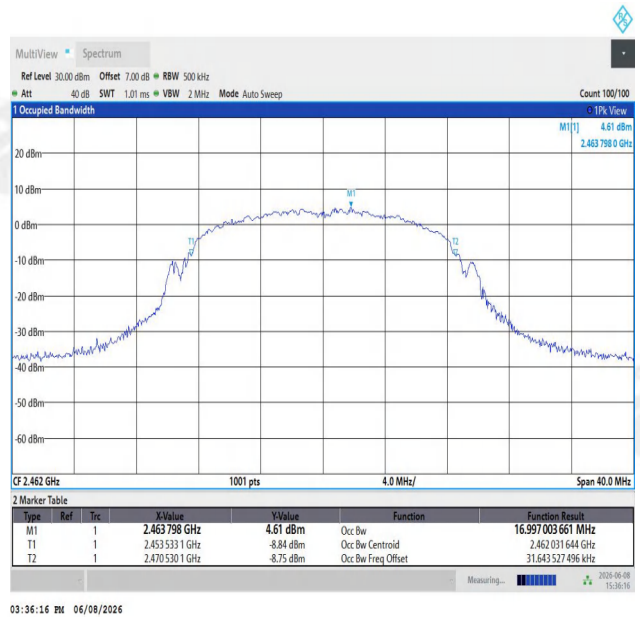
11G-Ant1-2462
