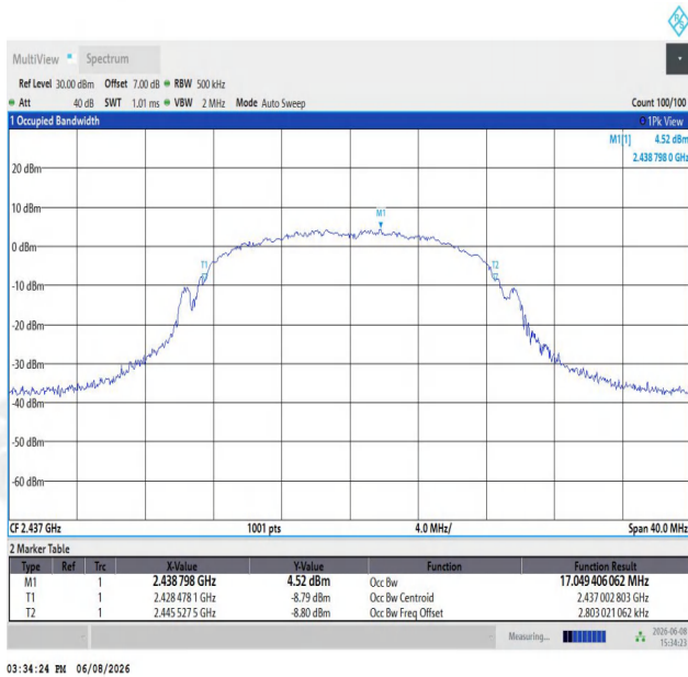
11G-Ant1-2437
