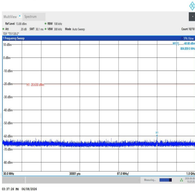
11G-Ant1-2462-30~1000-PASS
