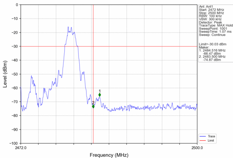
2M_HCH_2480MHz_Ant1_NTNV
