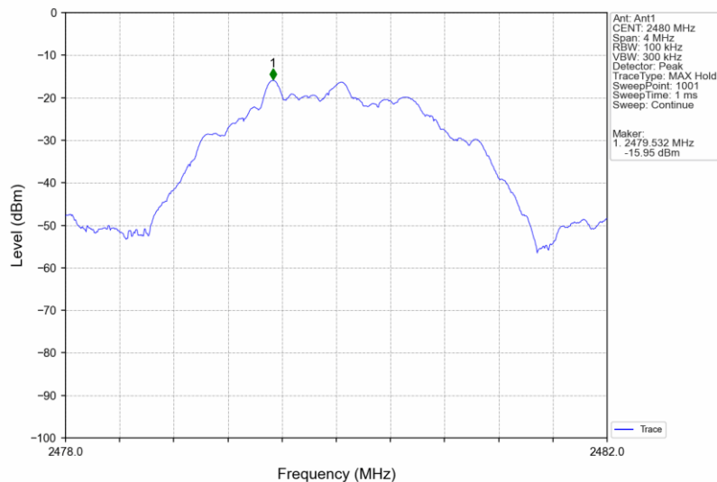
2M_HCH_2480MHz_Ant1_NTNV
