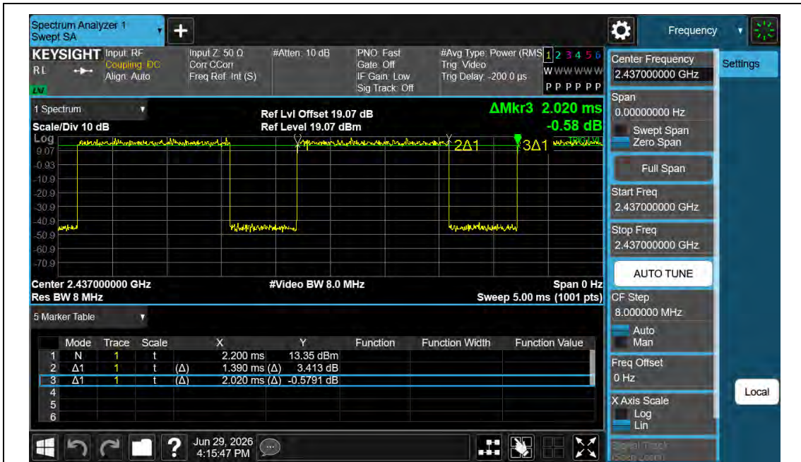
NTNV-11G-Ant1-2437
