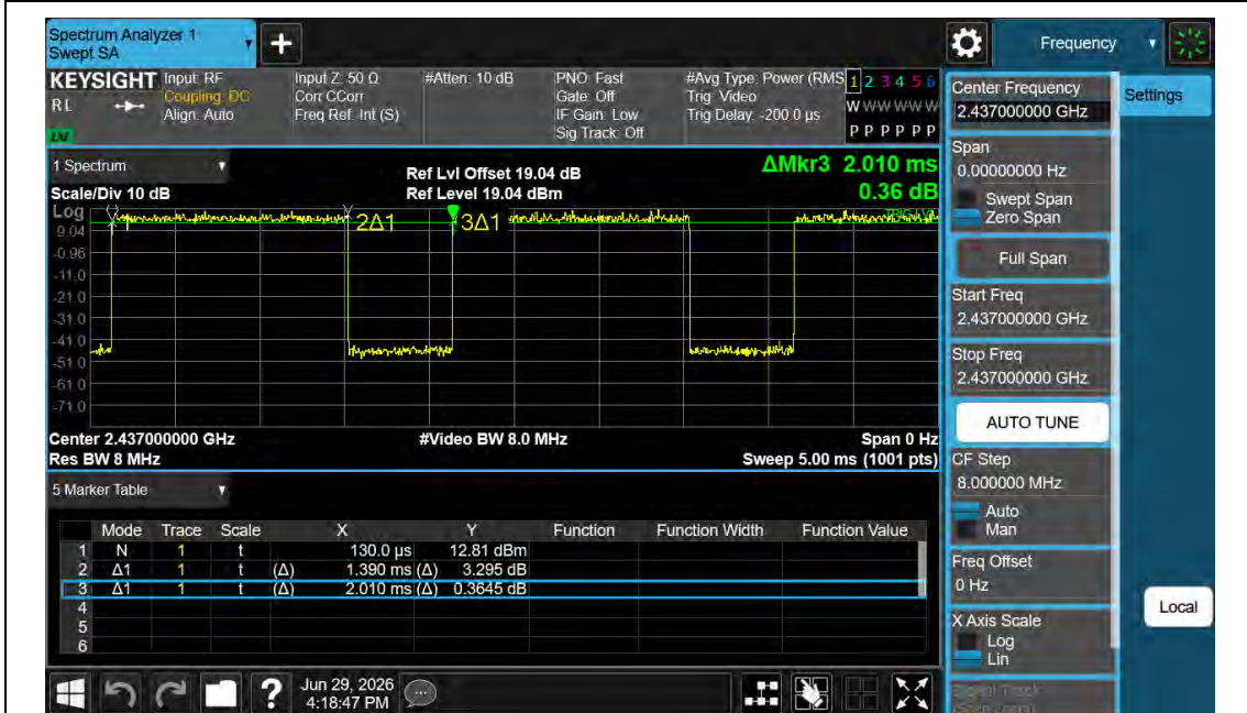
NTNV-11N20MIMO-Ant0-2437
