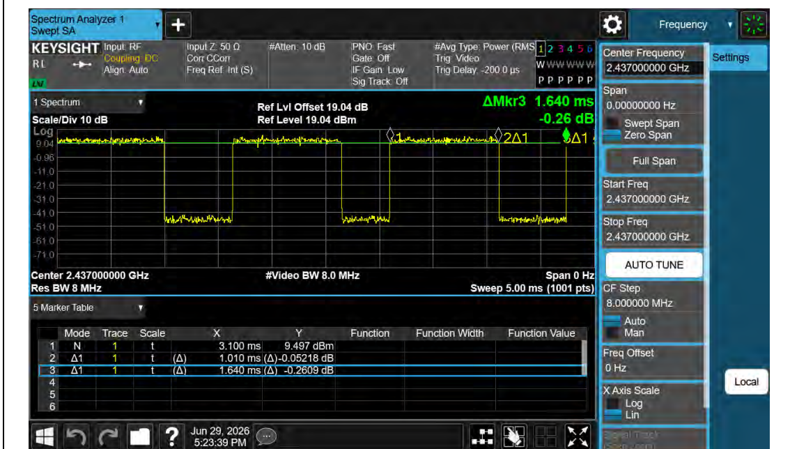
NTNV-11AX40MIMO-Ant0-2437
