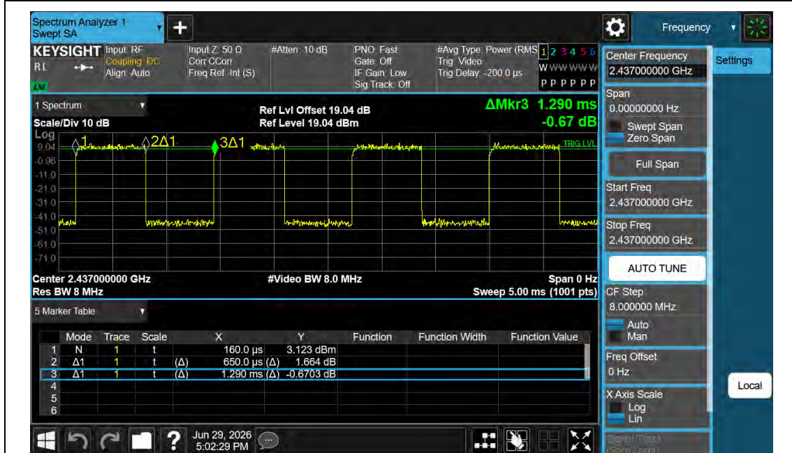
NTNV-11AX20MIMO-Ant0-2437
