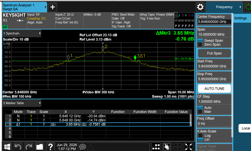
FSK-Ant1-5848
