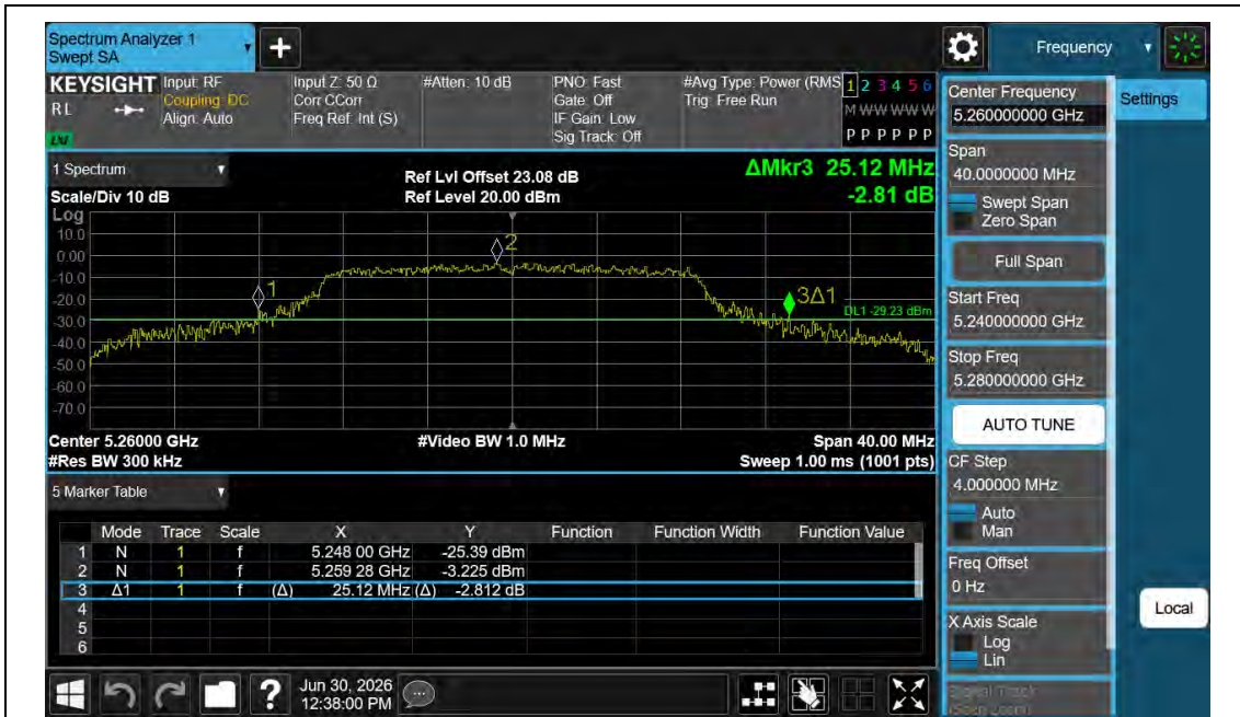
11N20MIMO-Ant1-5260
