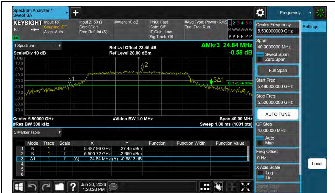
11N20MIMO-Ant1-5500
