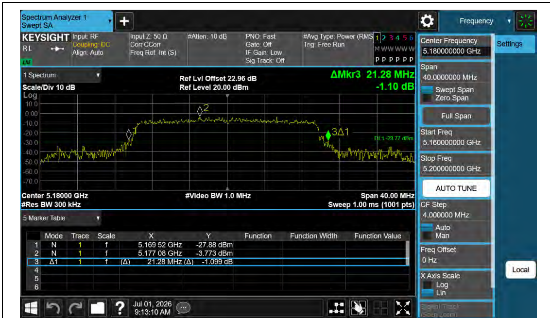
11AX20MIMO-Ant1-5180
