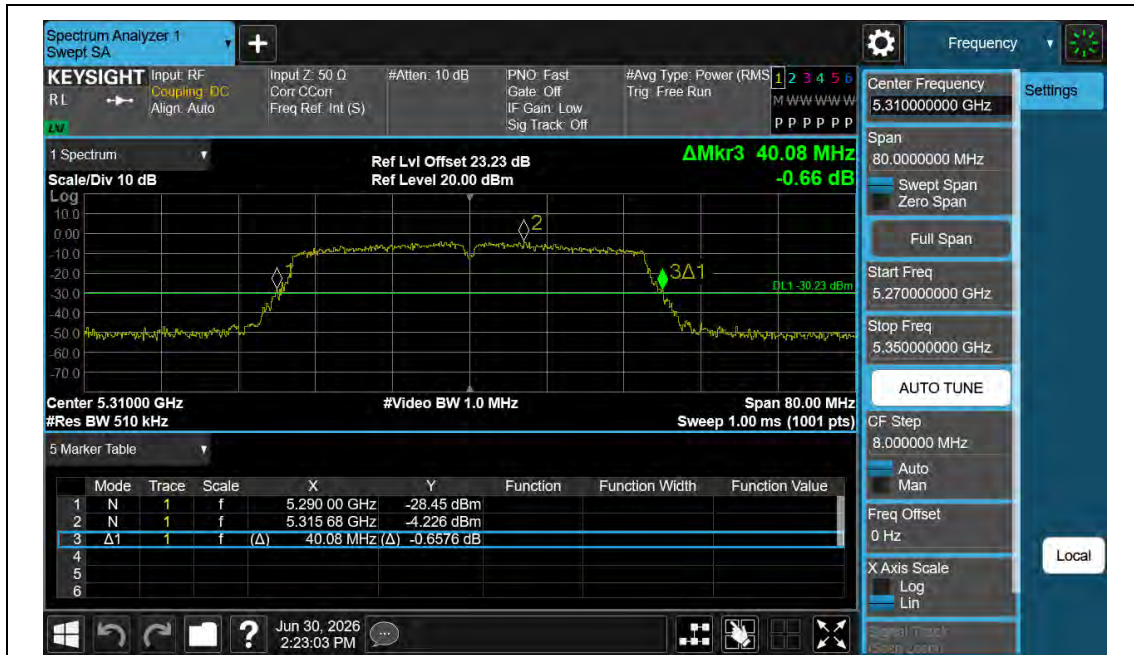
11N40MIMO-Ant1-5310
