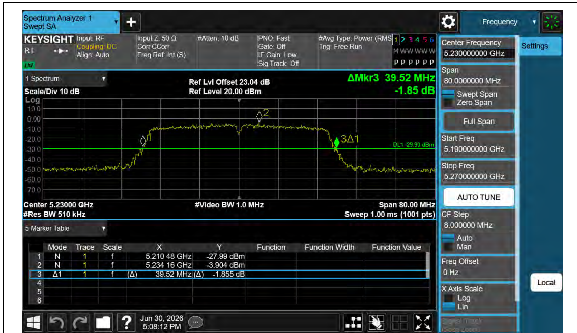
11AC40MIMO-Ant1-5230
