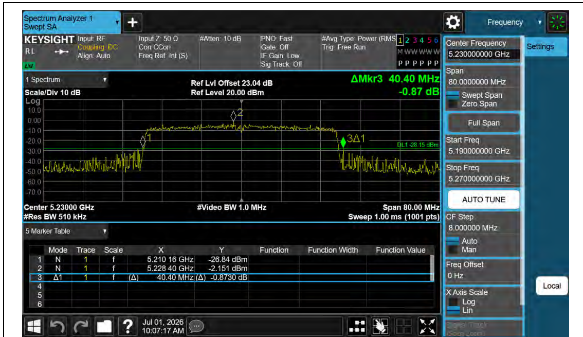
11AX40MIMO-Ant1-5230
