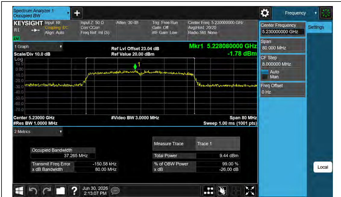
11N40MIMO-Ant1-5230
