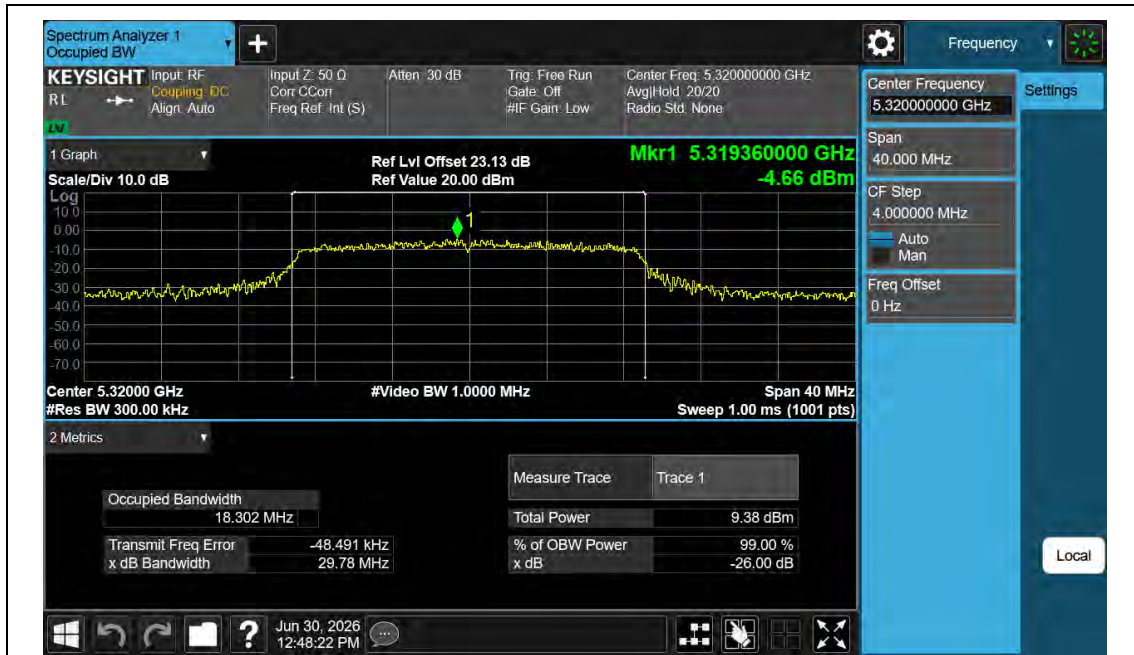
11N20MIMO-Ant1-5320
