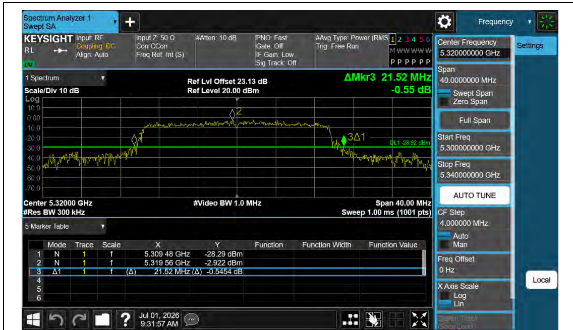
11AX20MIMO-Ant1-5320
