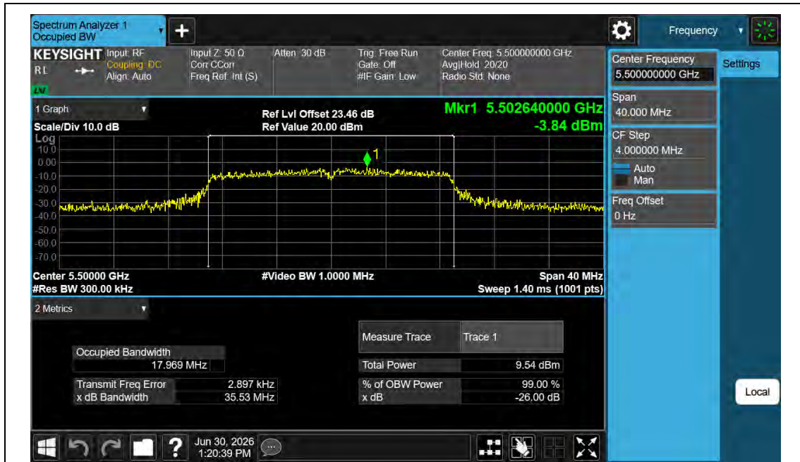
11N20MIMO-Ant1-5500
