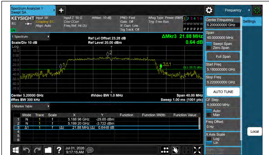
11AX20MIMO-Ant1-5200
