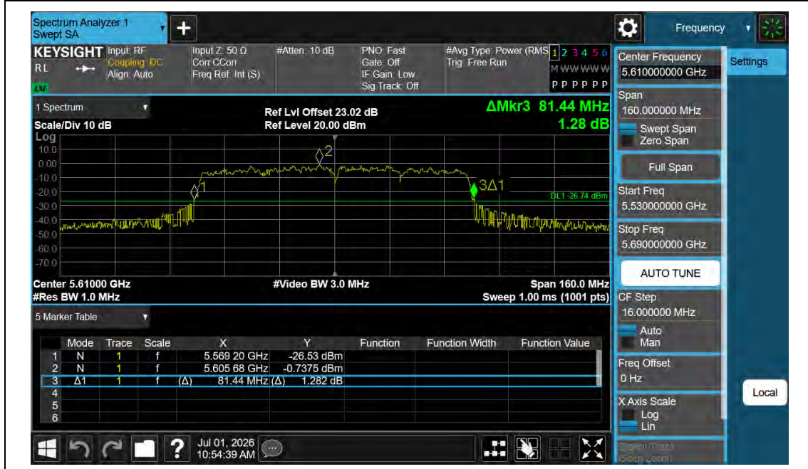
11AX80MIMO-Ant1-5610
