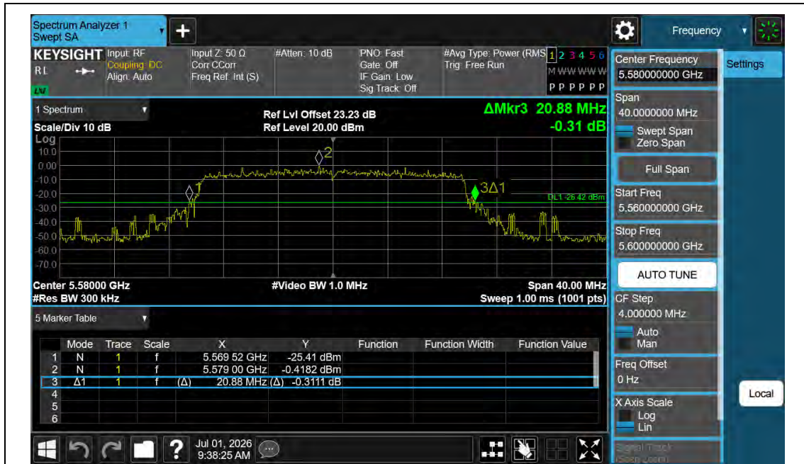
11AX20MIMO-Ant1-5580
