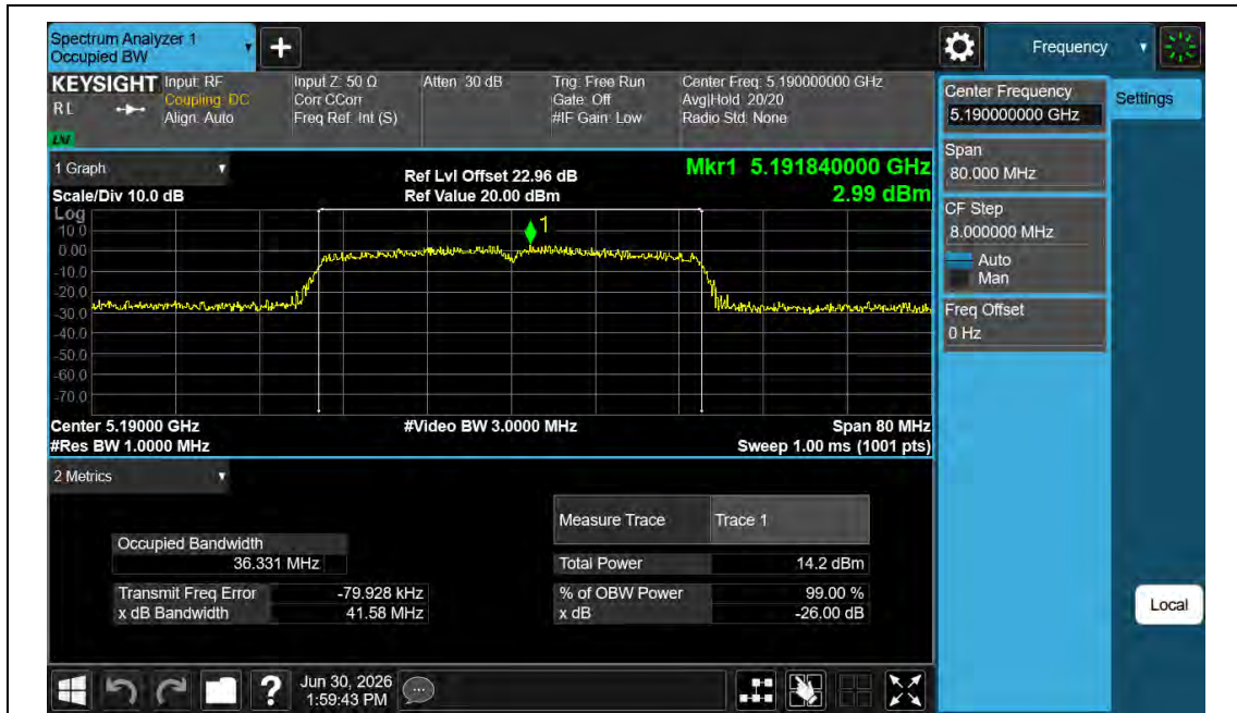
11N40MIMO-Ant1-5190
