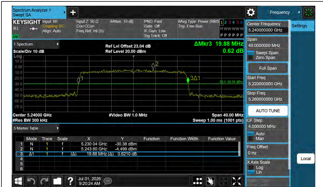
11AX20MIMO-Ant1-5240
