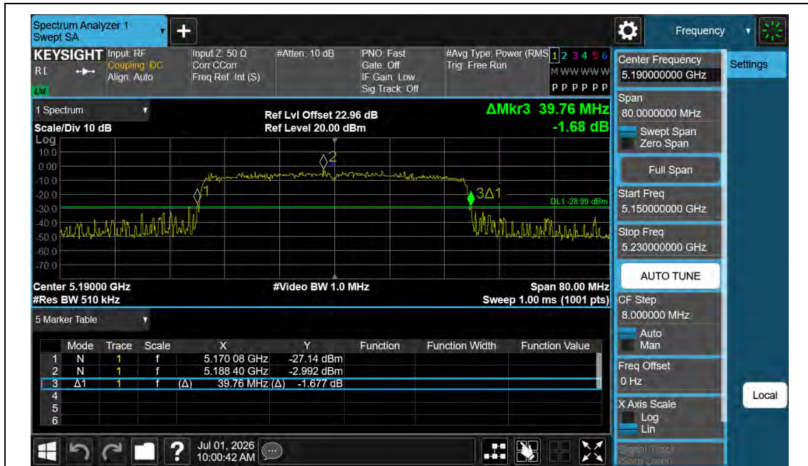
11AX40MIMO-Ant1-5190
