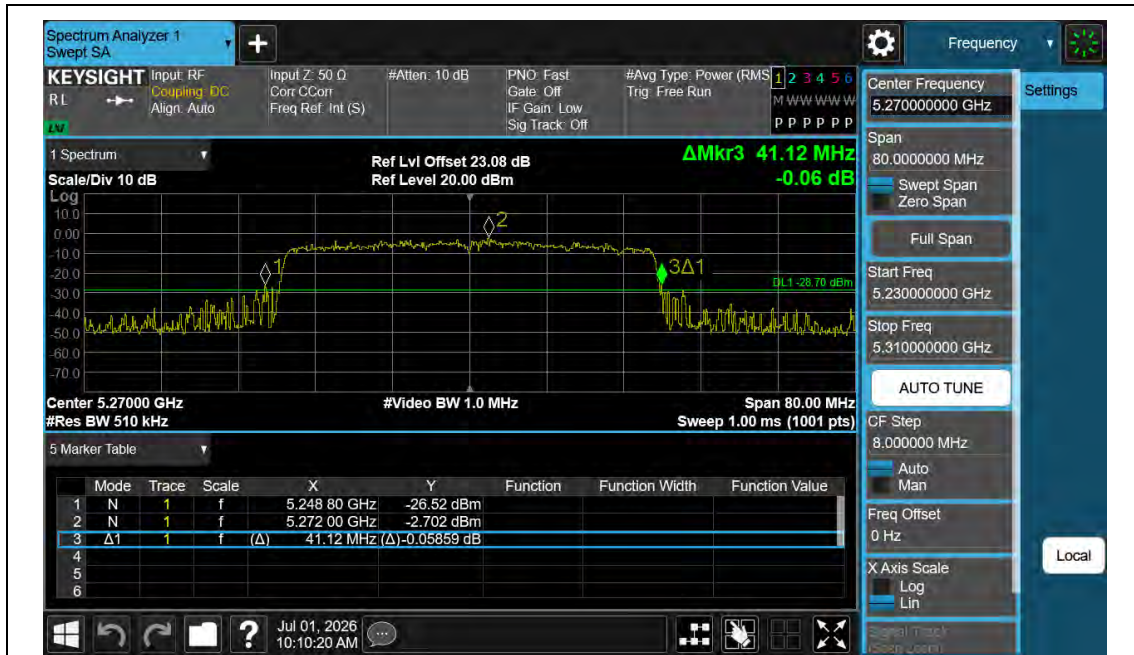
11AX40MIMO-Ant1-5270
