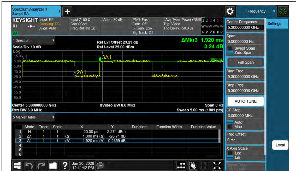
NTNV-11N20MIMO-Ant1-5300
