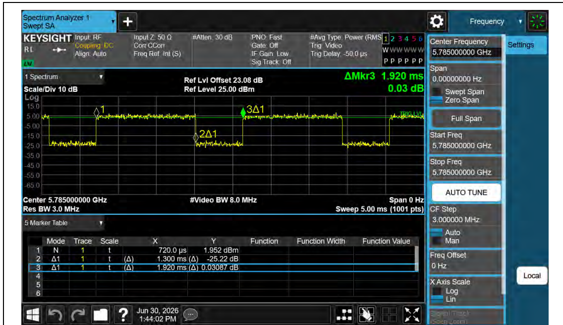
NTNV-11N20MIMO-Ant1-5785
