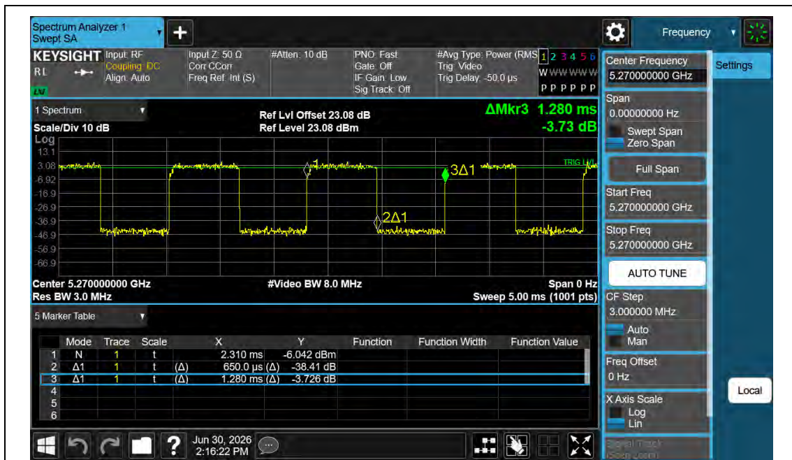
NTNV-11N40MIMO-Ant1-5270
