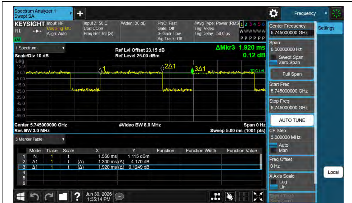
NTNV-11N20MIMO-Ant1-5745
