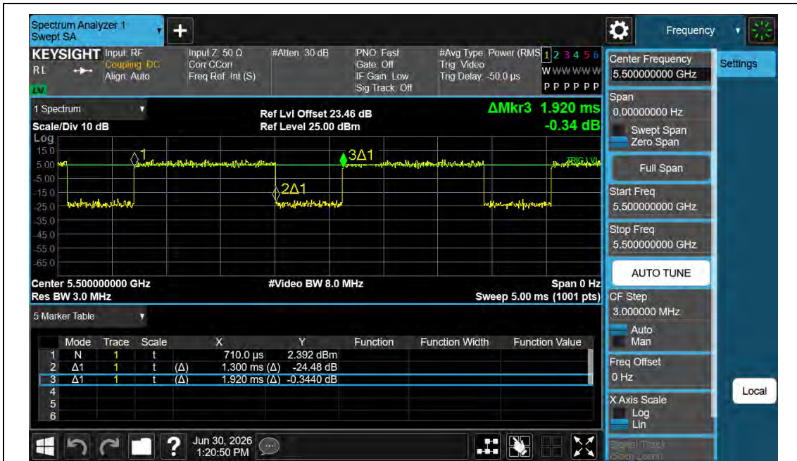
NTNV-11N20MIMO-Ant1-5500
