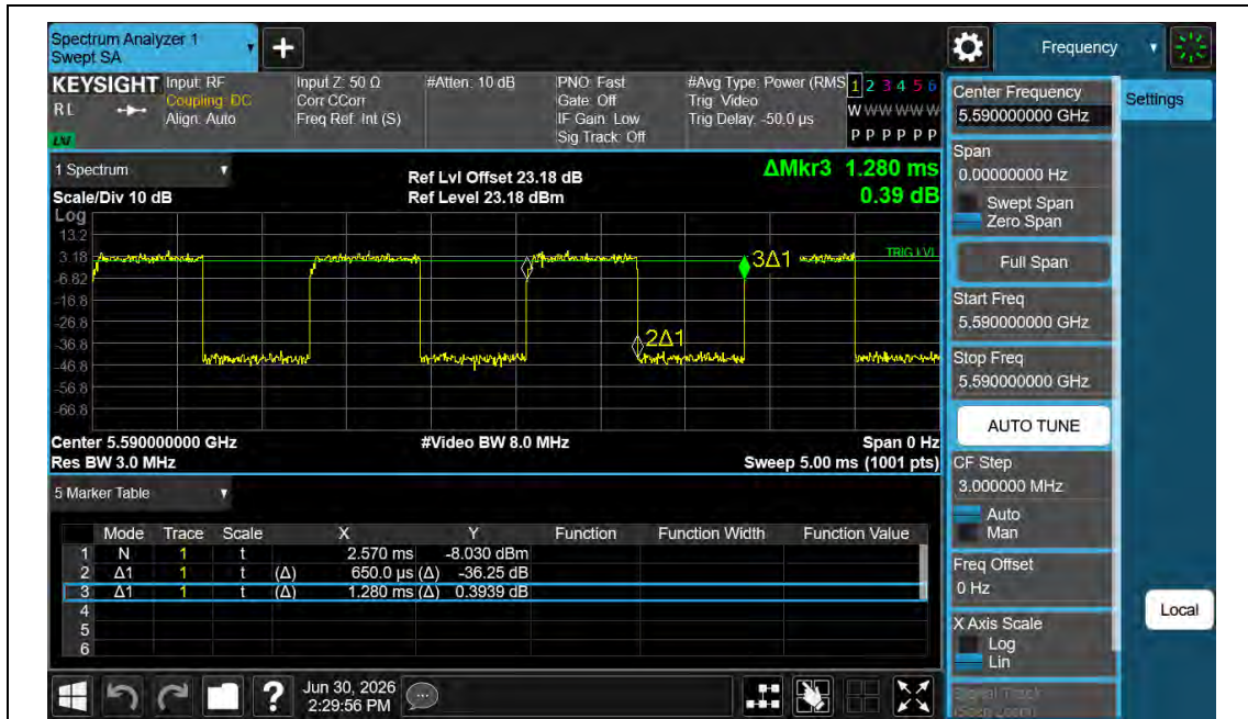
NTNV-11N40MIMO-Ant1-5590
