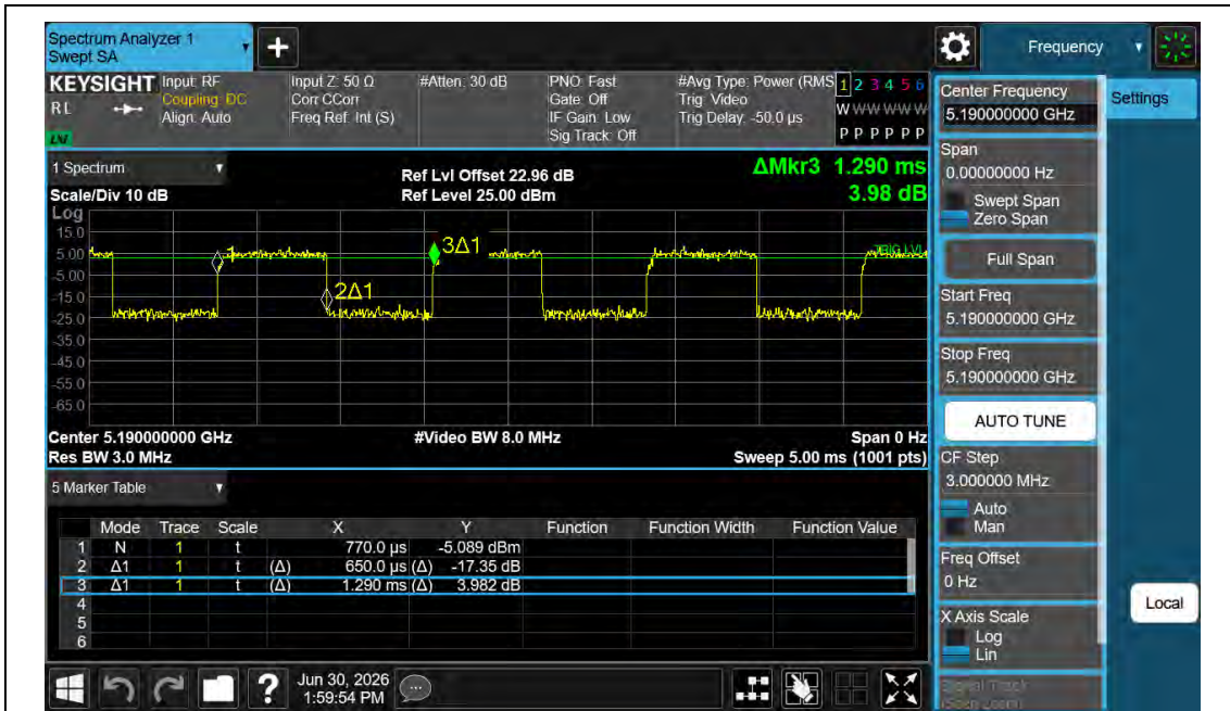
NTNV-11N40MIMO-Ant1-5190
