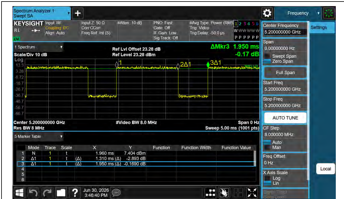
NTNV-11AC20MIMO-Ant1-5200
