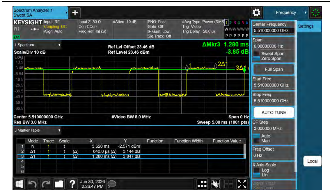
NTNV-11N40MIMO-Ant1-5510
