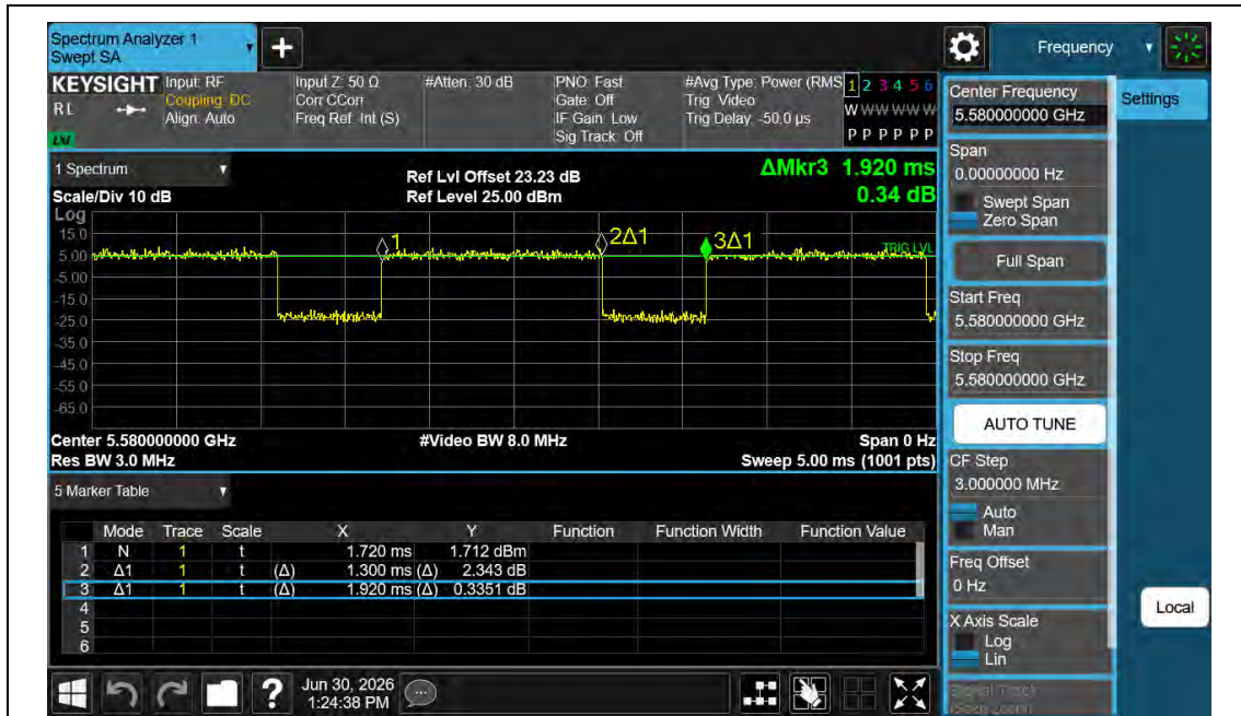
NTNV-11N20MIMO-Ant1-5580
