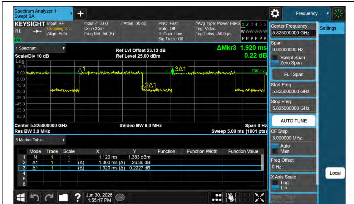
NTNV-11N20MIMO-Ant1-5825
