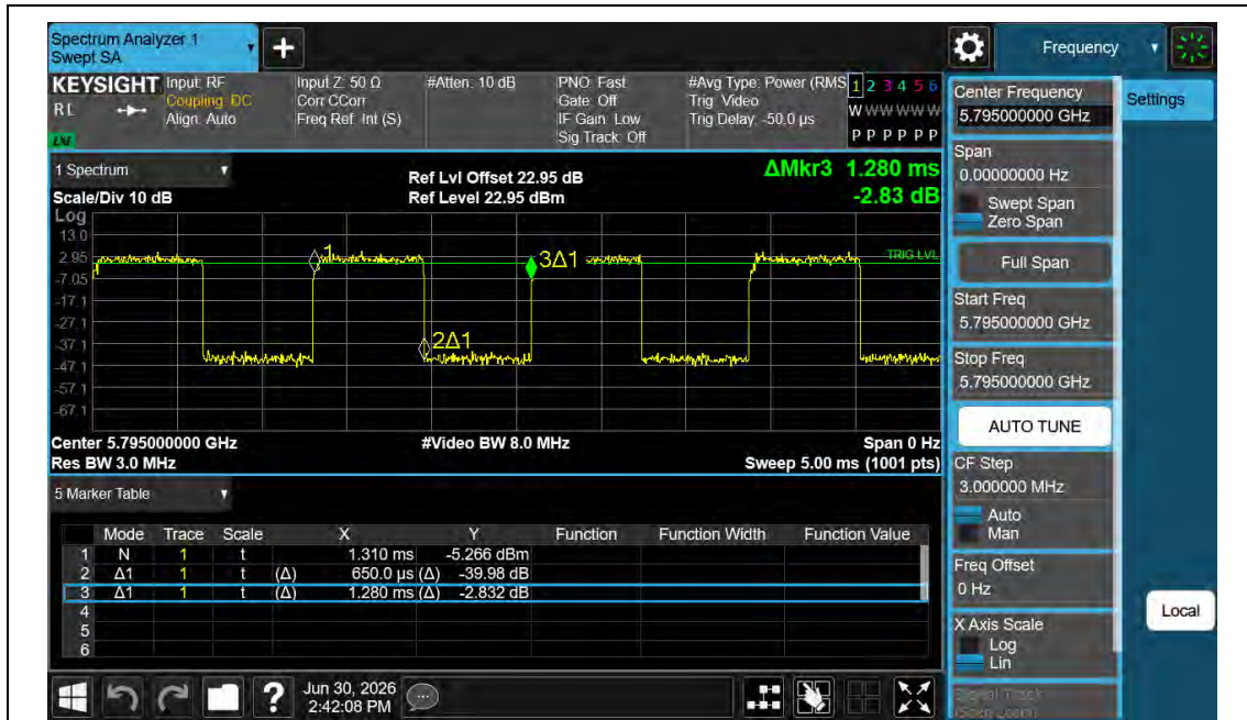
NTNV-11N40MIMO-Ant1-5795
