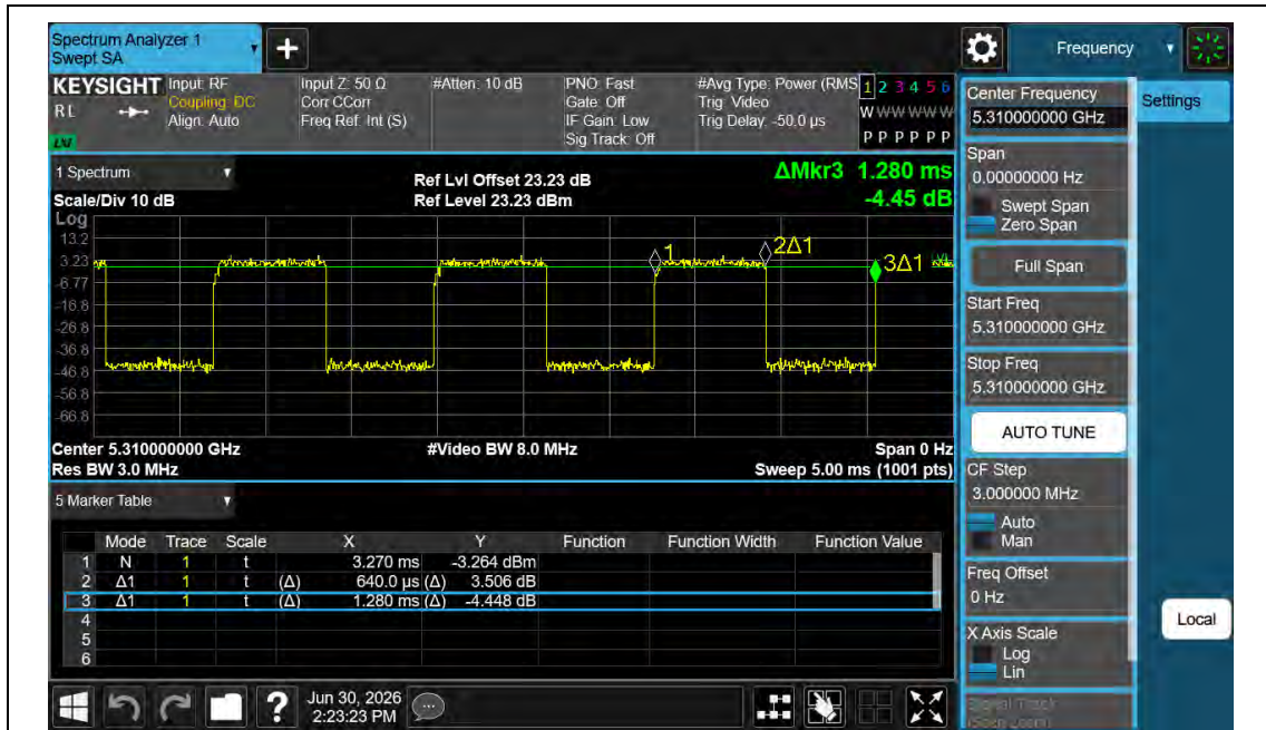
NTNV-11N40MIMO-Ant1-5310
