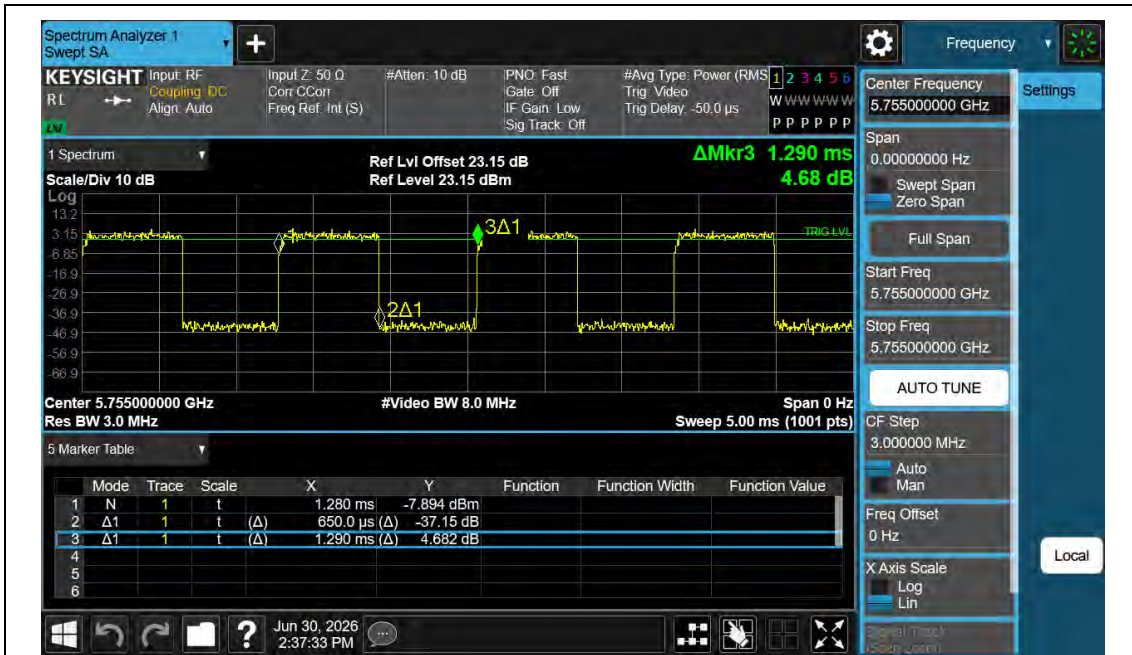
NTNV-11N40MIMO-Ant1-5755
