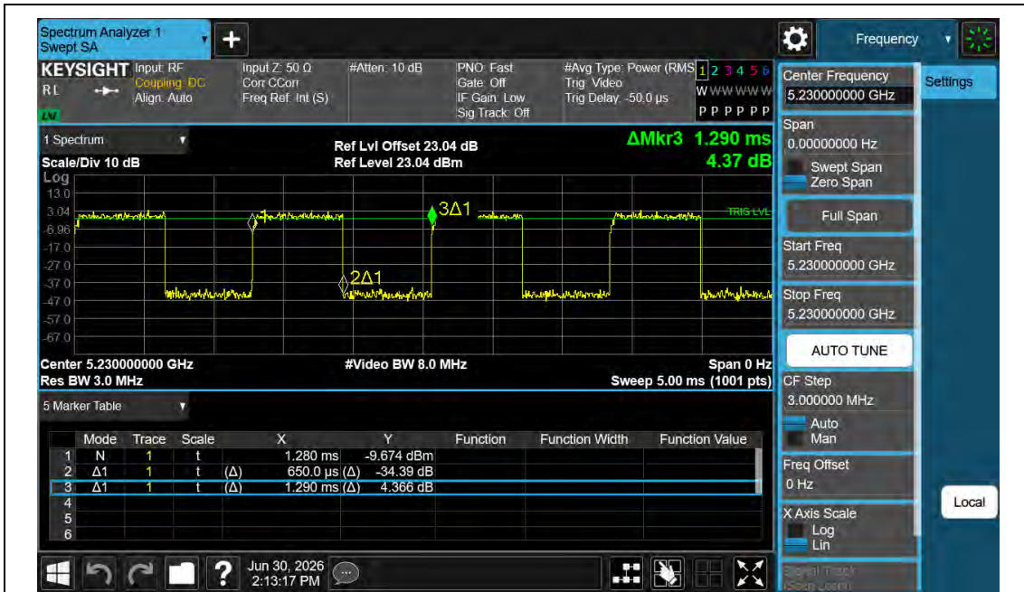
NTNV-11N40MIMO-Ant1-5230
