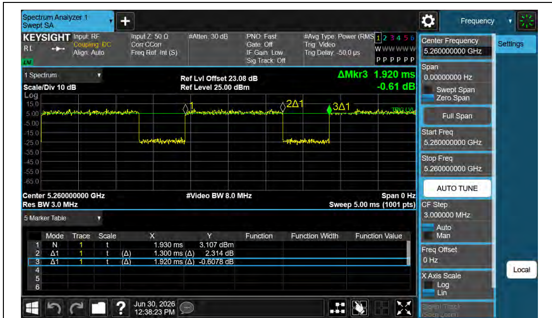
NTNV-11N20MIMO-Ant1-5260
