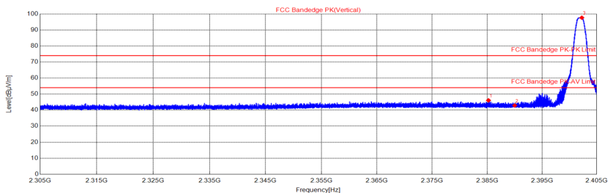
BLE_1M_2402_Ant1/ Vertical
