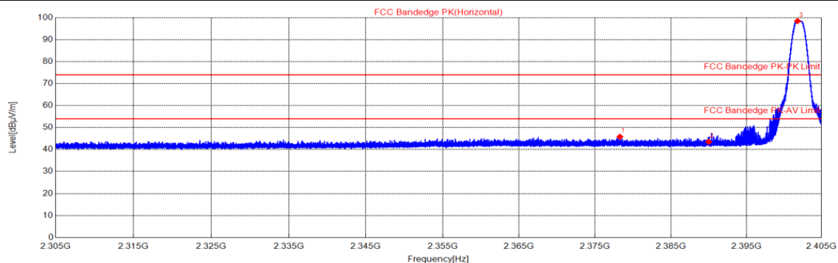
BLE_1M_2402_Ant1/ Horizontal
