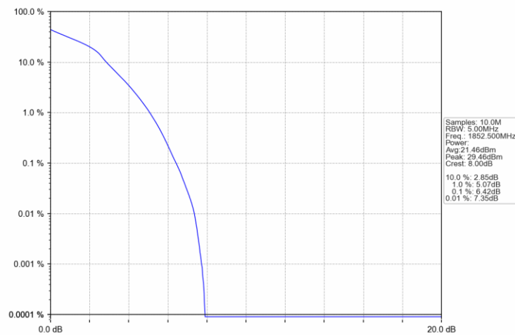
Band2 5MHz 16QAM LCH 1852.5MHz RB 25 0 NTV
