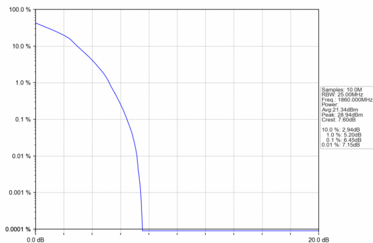
Band2 20MHz 16QAM LCH 1860MHz RB 27 0 NTNV
