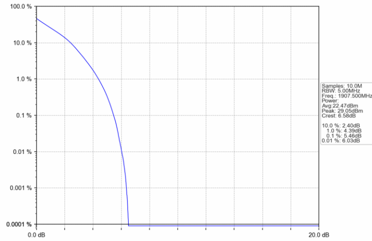
Band2 5MHz QPSK HCH 1907.5MHz RB 25 0 NTV
