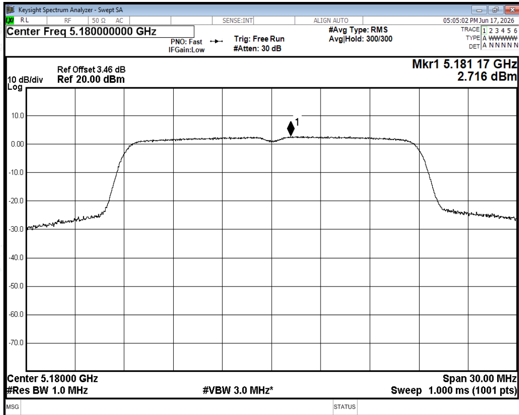
PSD NVNT ac20 5180MHz Ant0
