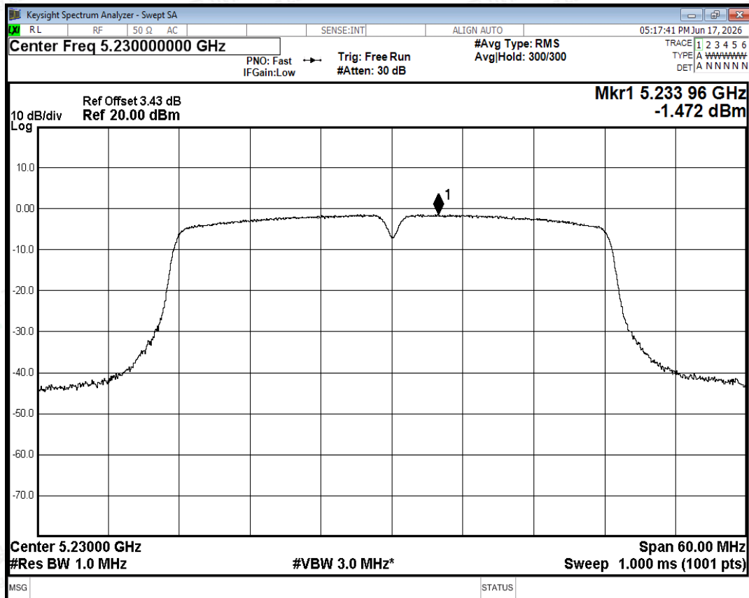
PSD NVNT n40 5230MHz Ant0
