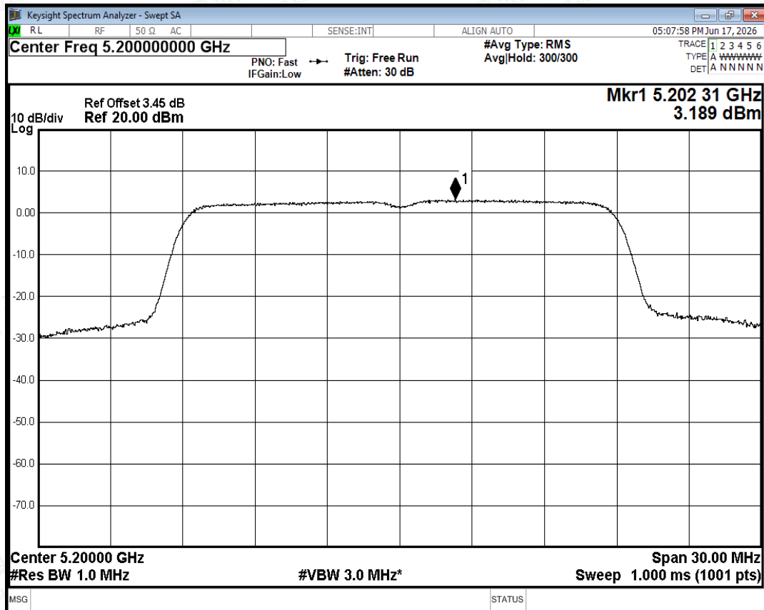
PSD NVNT ac20 5200MHz Ant0
