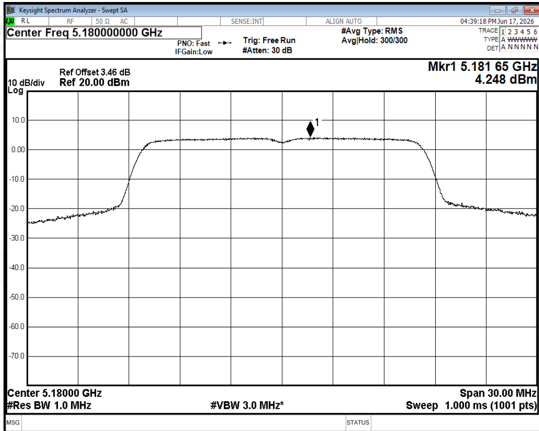
PSD NVNT a 5180MHz Ant0
