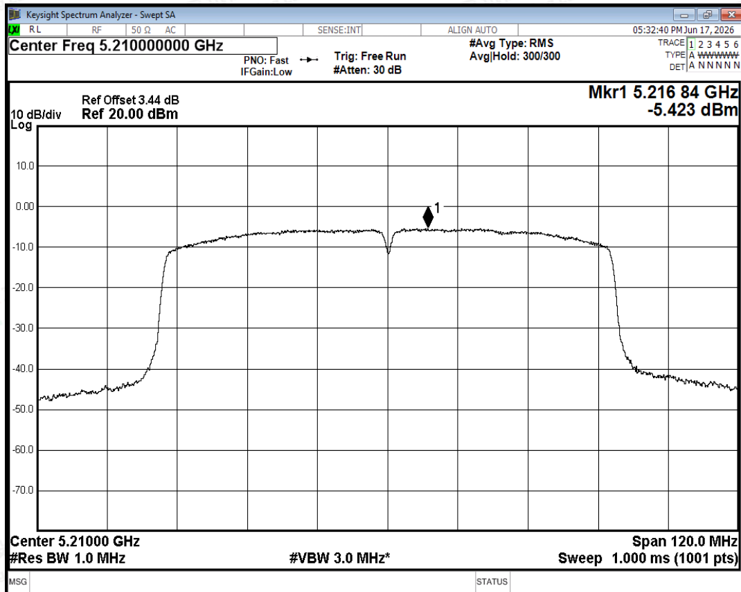
PSD NVNT ac80 5210MHz Ant0
