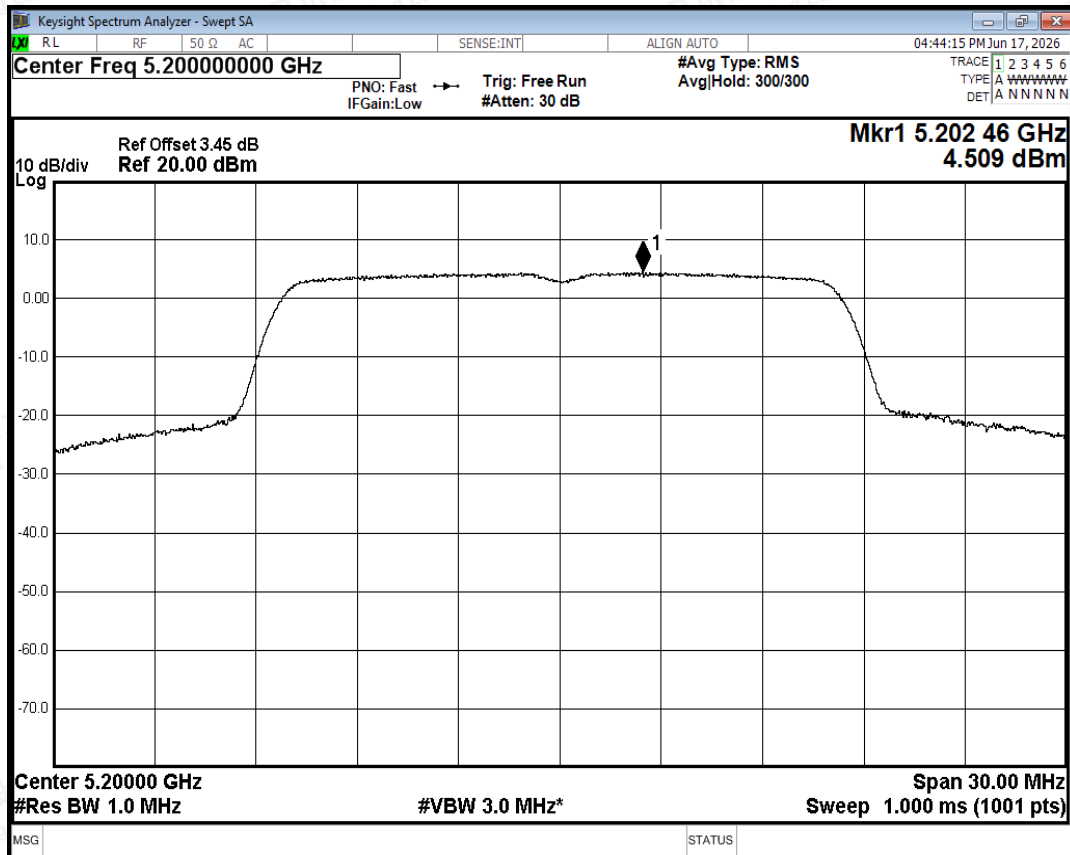
PSD NVNT a 5200MHz Ant0
