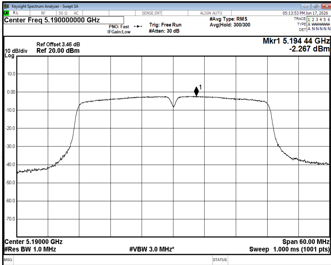
PSD NVNT n40 5190MHz Ant0
