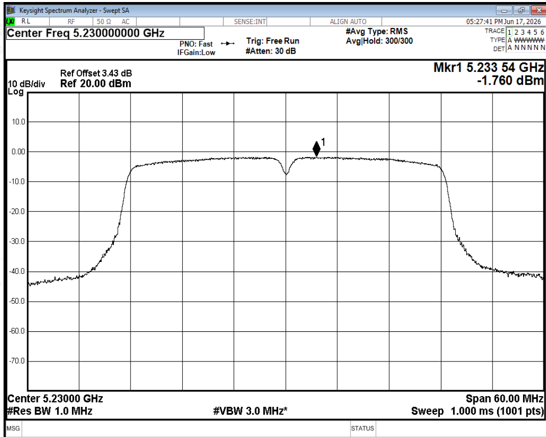
PSD NVNT ac40 5230MHz Ant0
