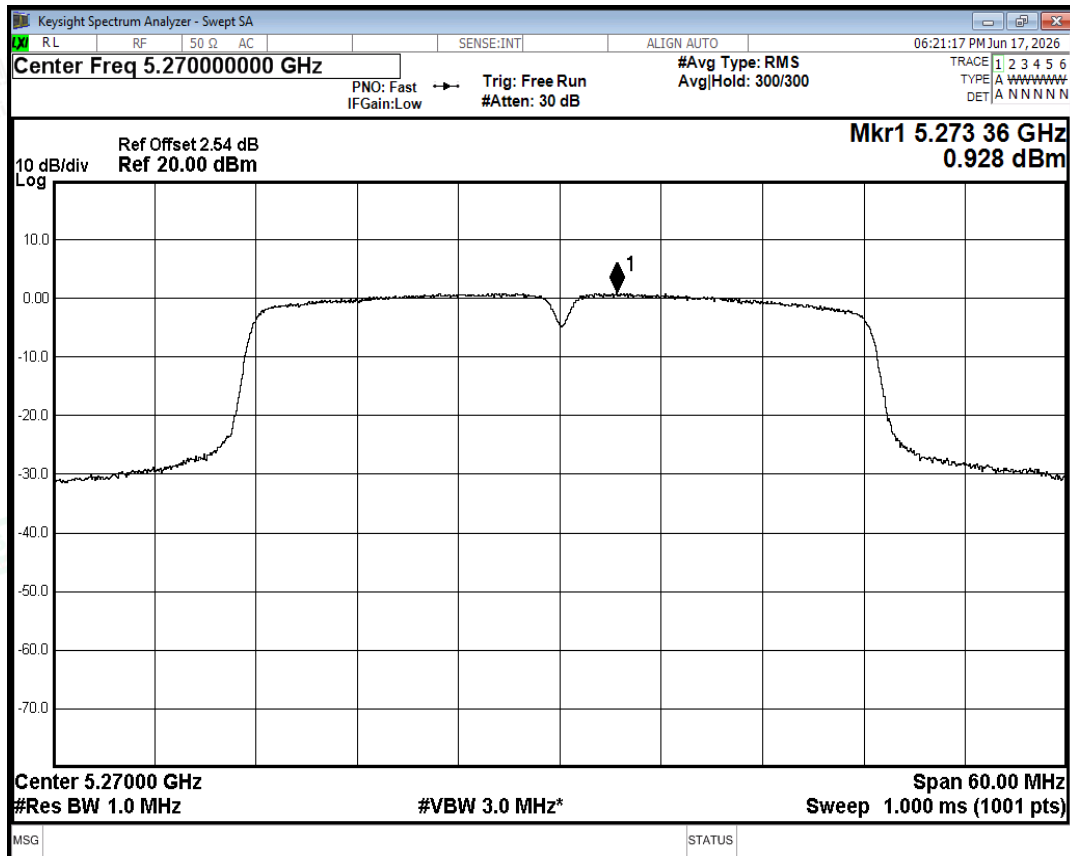
PSD NVNT n40 5270MHz Ant0
