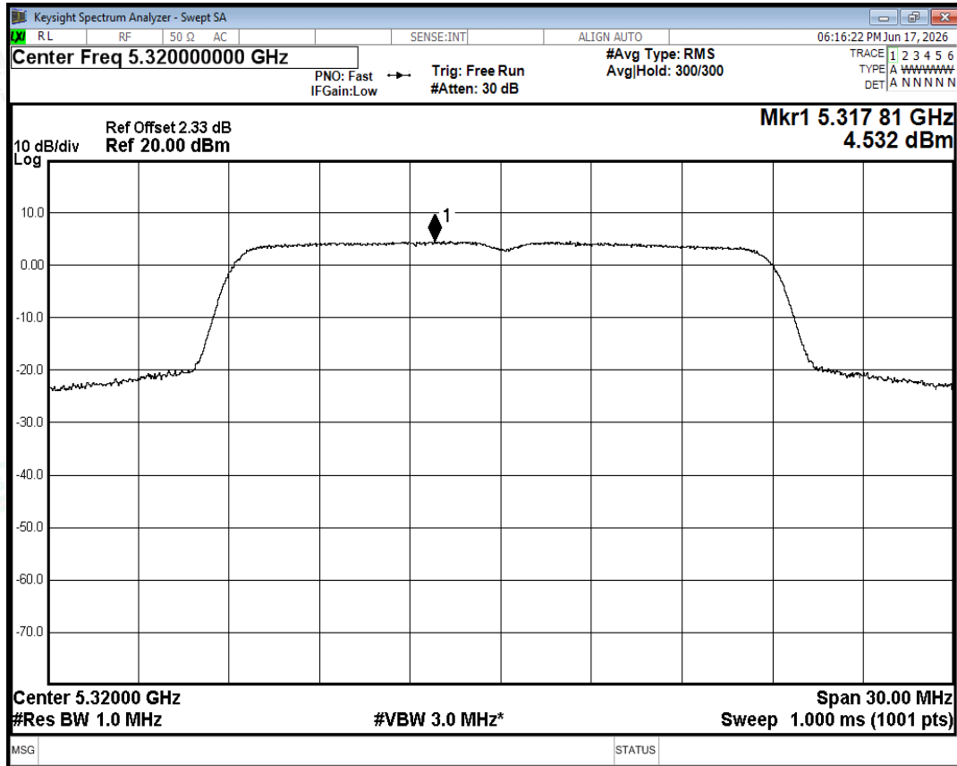
PSD NVNT ac20 5320MHz Ant0
