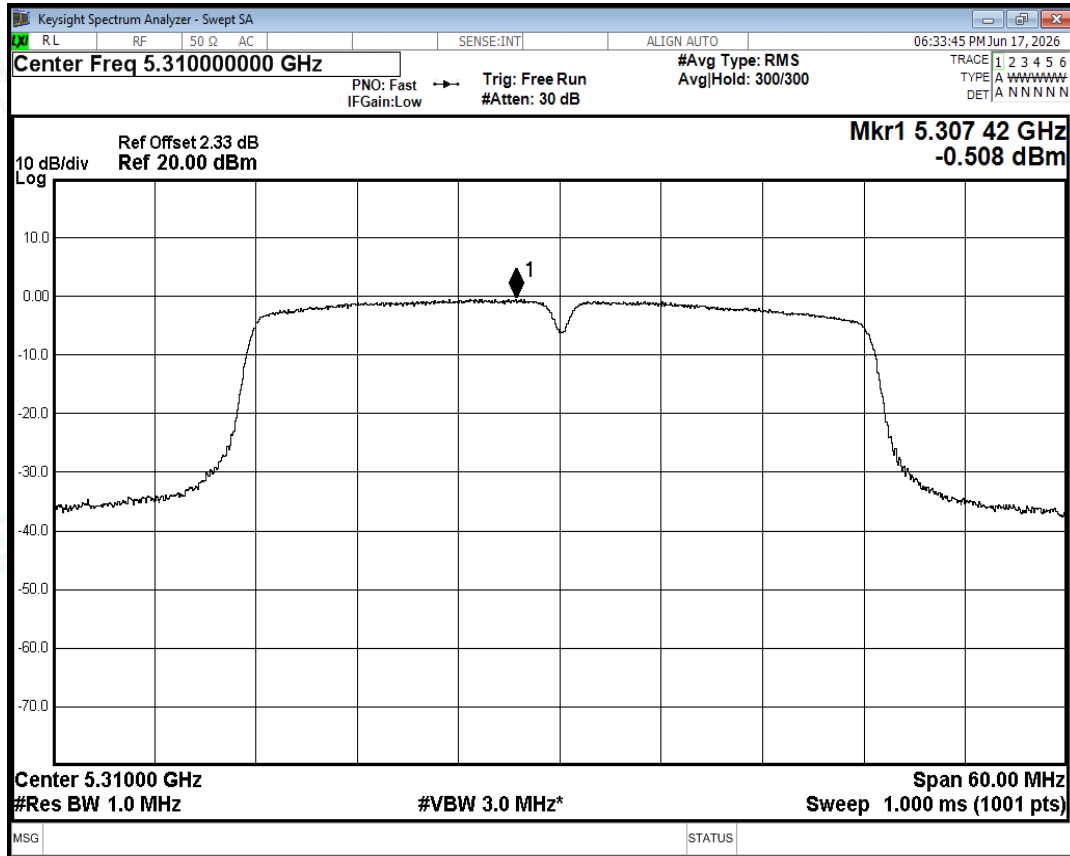
PSD NVNT ac40 5310MHz Ant0
