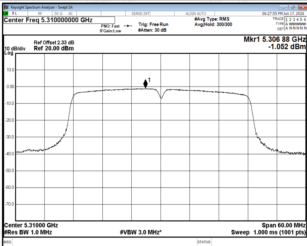
PSD NVNT n40 5310MHz Ant0
