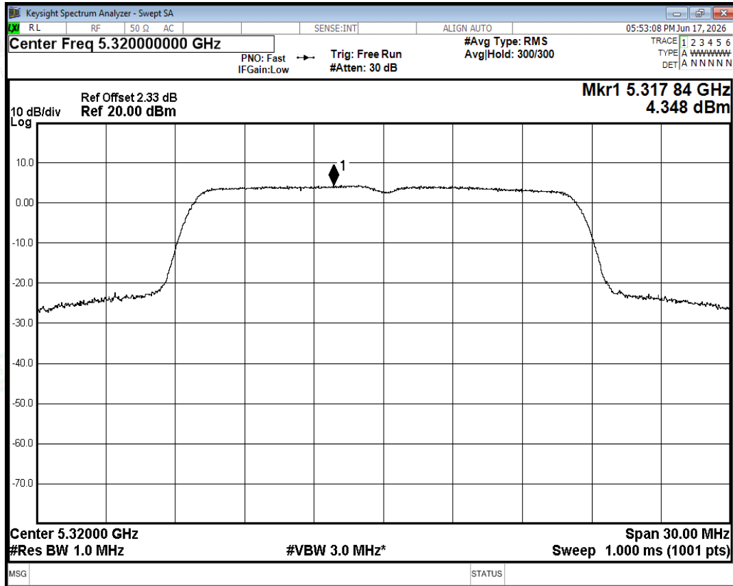
PSD NVNT a 5320MHz Ant0
