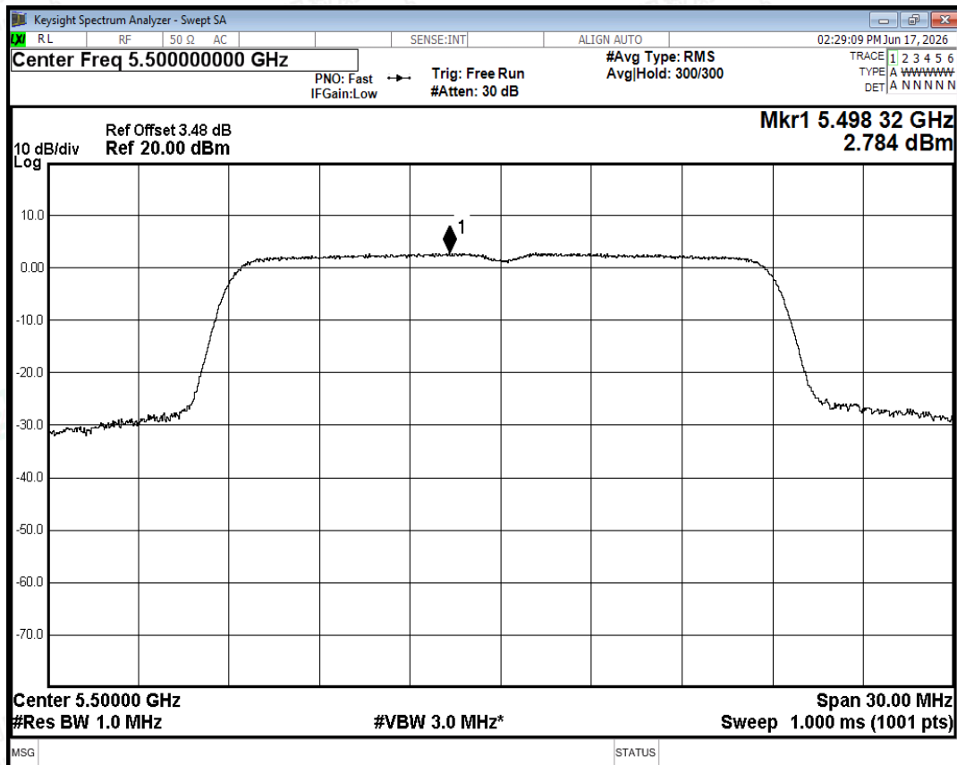
PSD NVNT ac20 5500MHz Ant0
