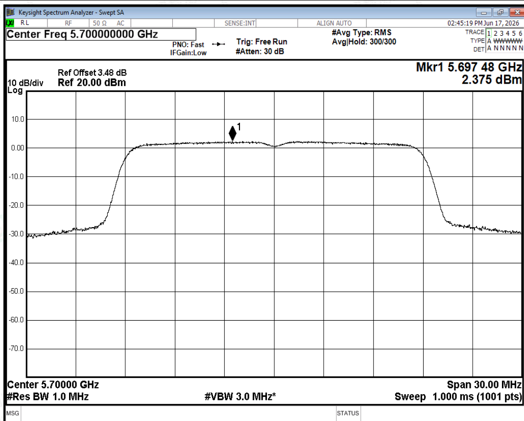
PSD NVNT ac20 5700MHz Ant0
