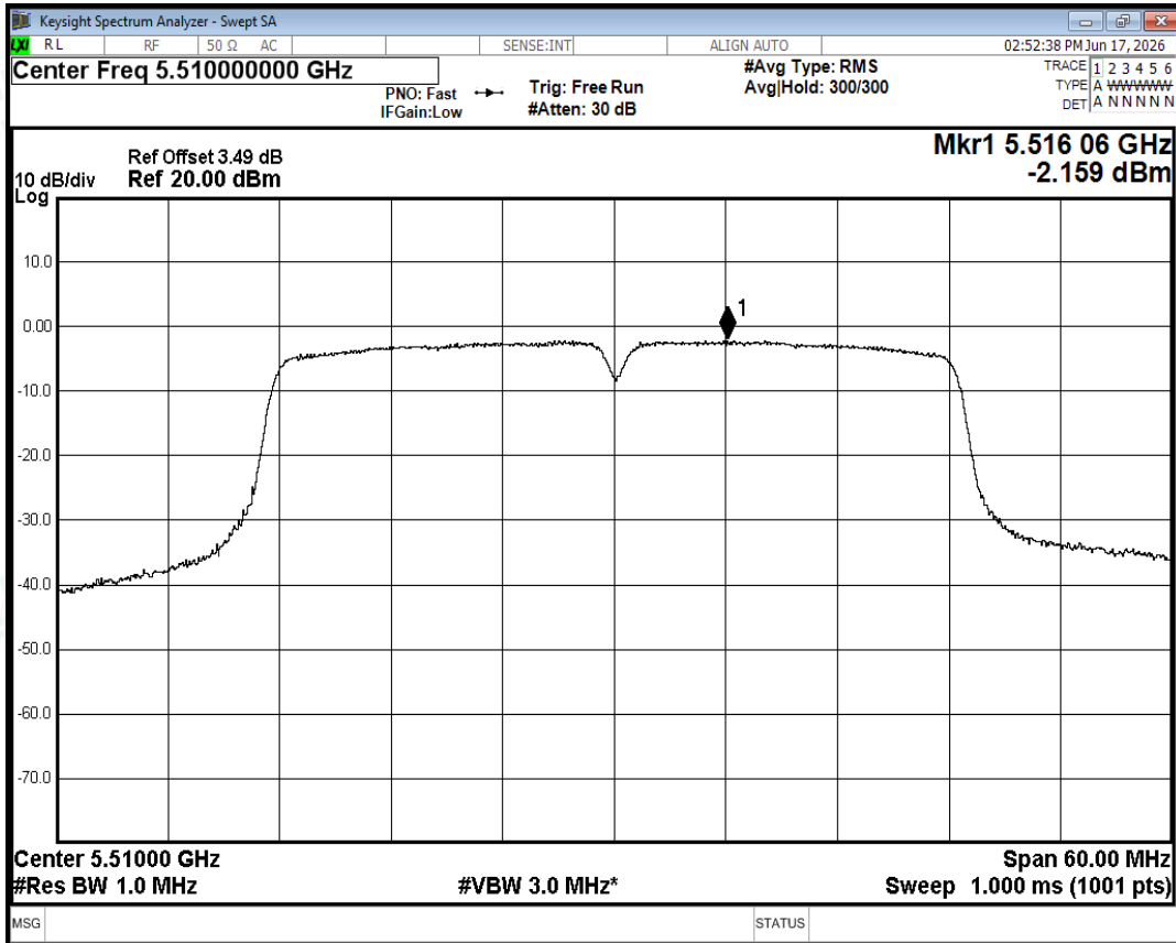
PSD NVNT n40 5510MHz Ant0
