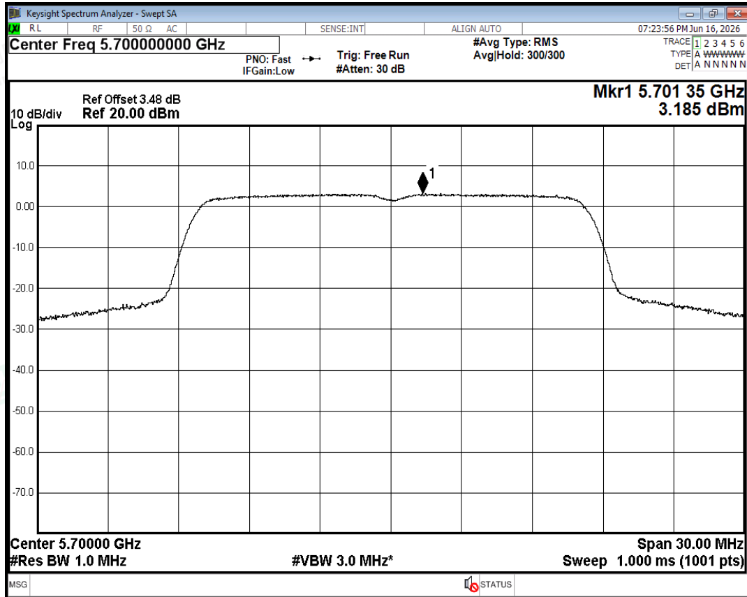
PSD NVNT a 5700MHz Ant0
