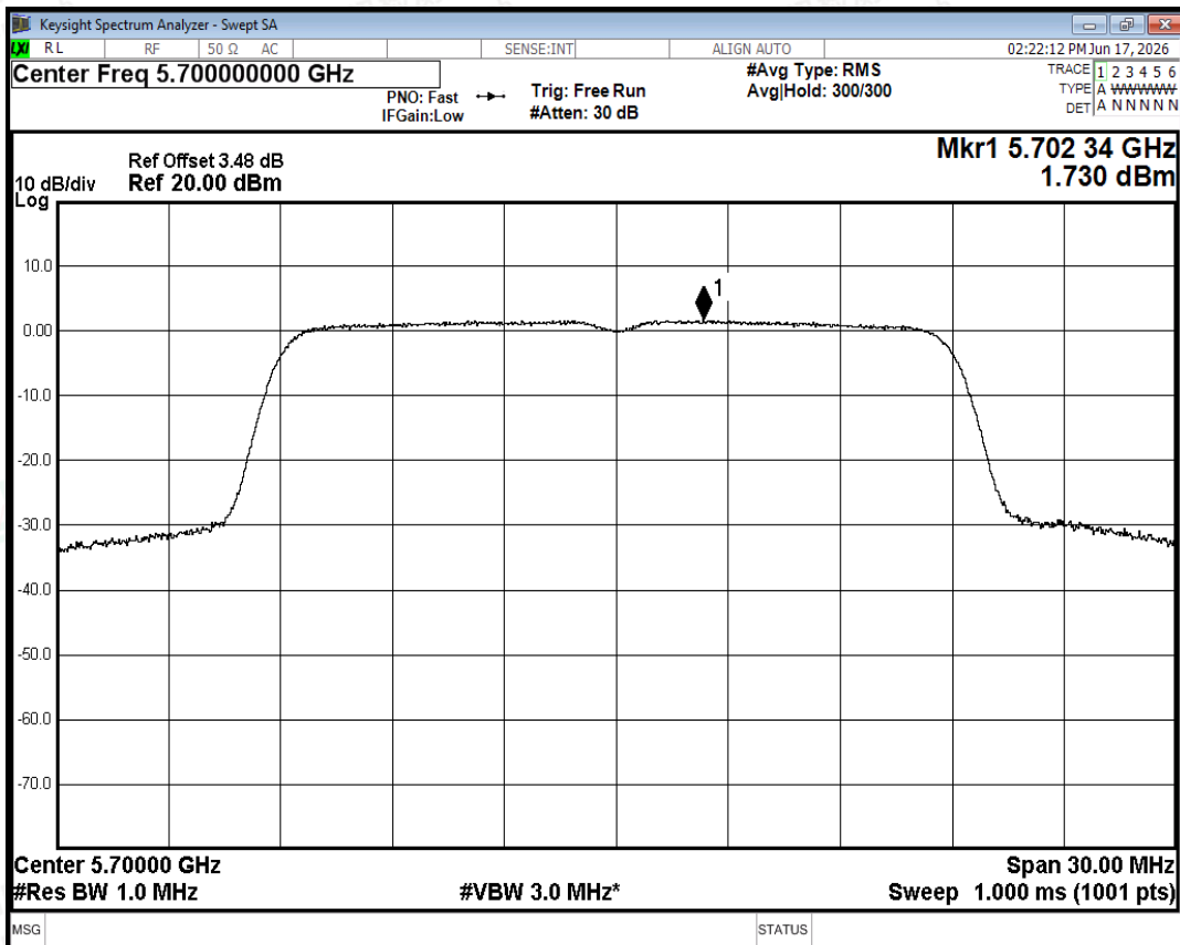
PSD NVNT n20 5700MHz Ant0
