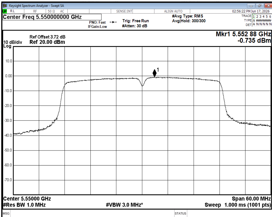
PSD NVNT n40 5550MHz Ant0
