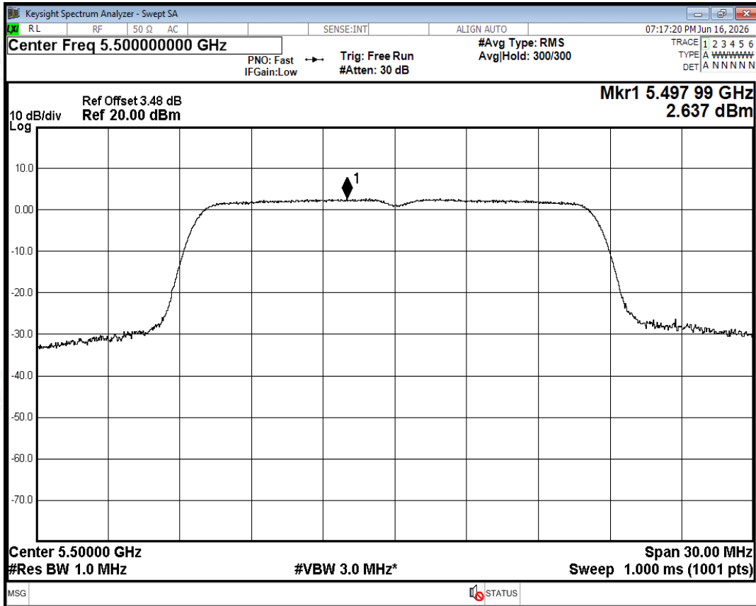
PSD NVNT a 5500MHz Ant0
