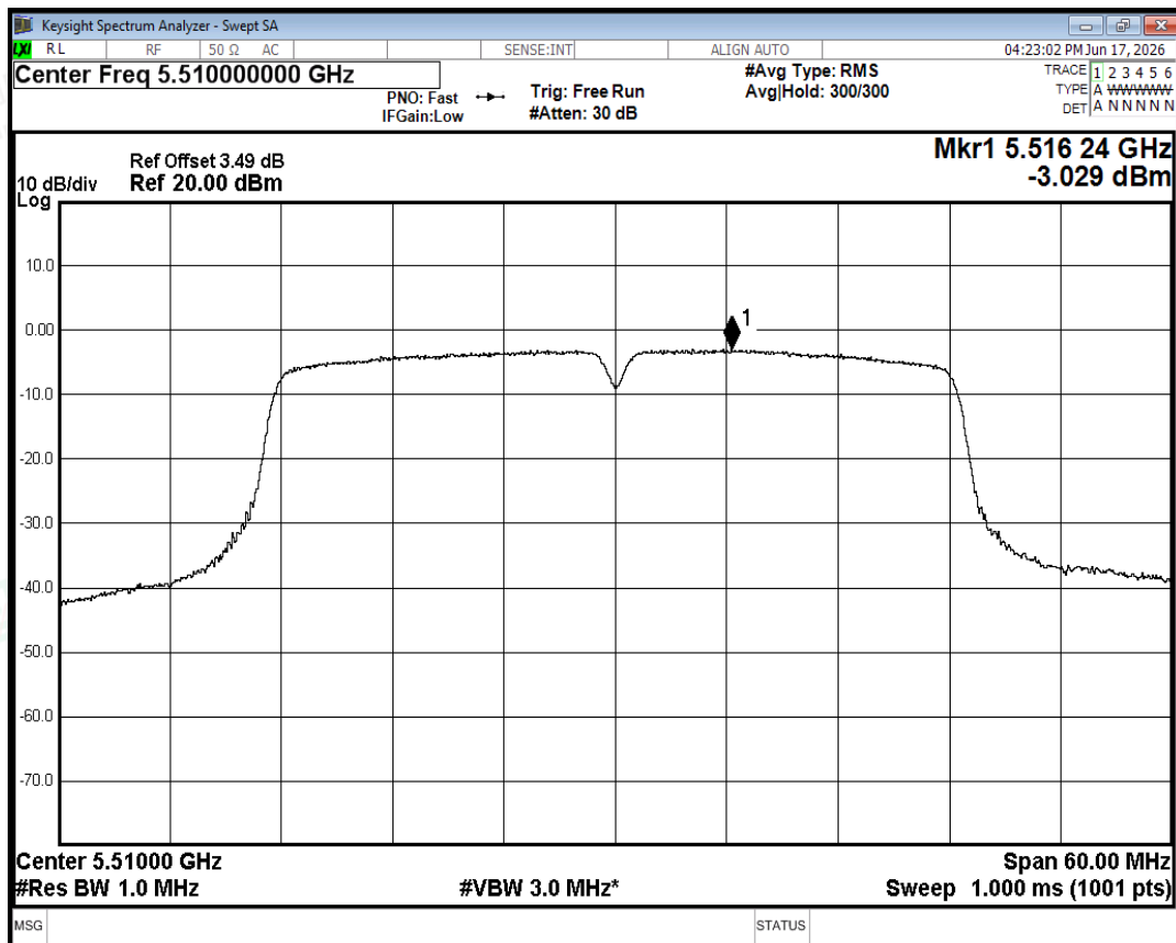
PSD NVNT ac40 5510MHz Ant0
