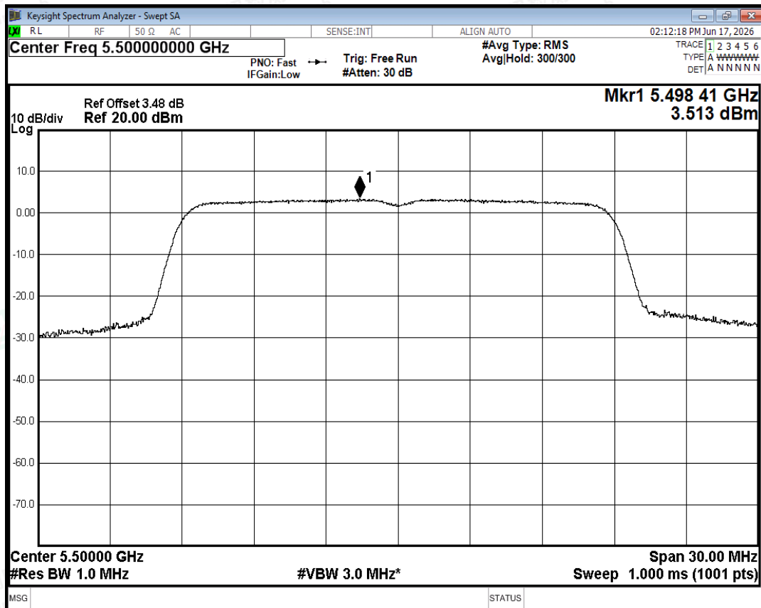
PSD NVNT n20 5500MHz Ant0
