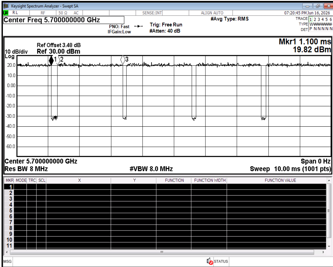
Duty Cycle NVNT a 5700MHz Ant0
