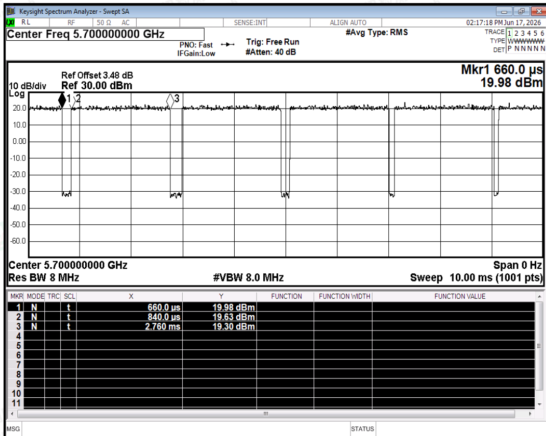
Duty Cycle NVNT n20 5700MHz Ant0
