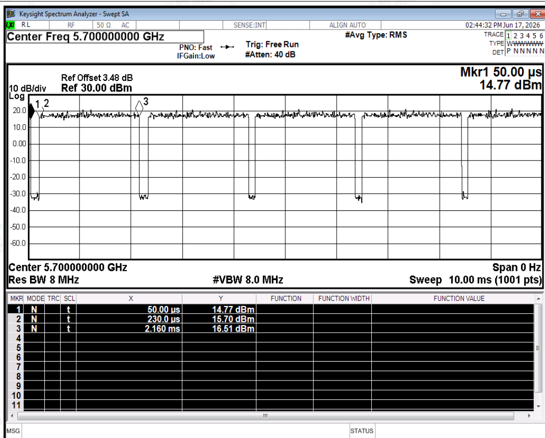
Duty Cycle NVNT ac20 5700MHz Ant0
