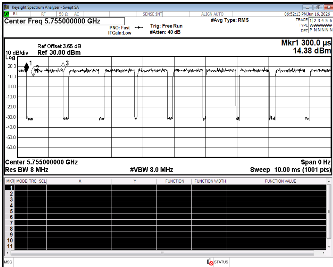
Duty Cycle NVNT n40 5755MHz Ant0
