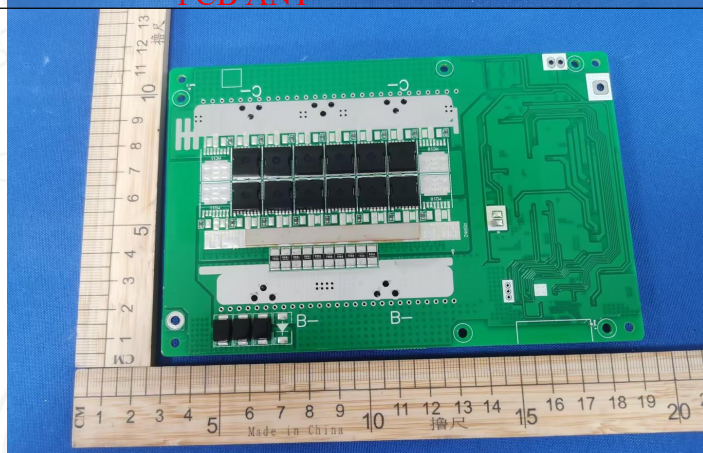
PCB ANT
