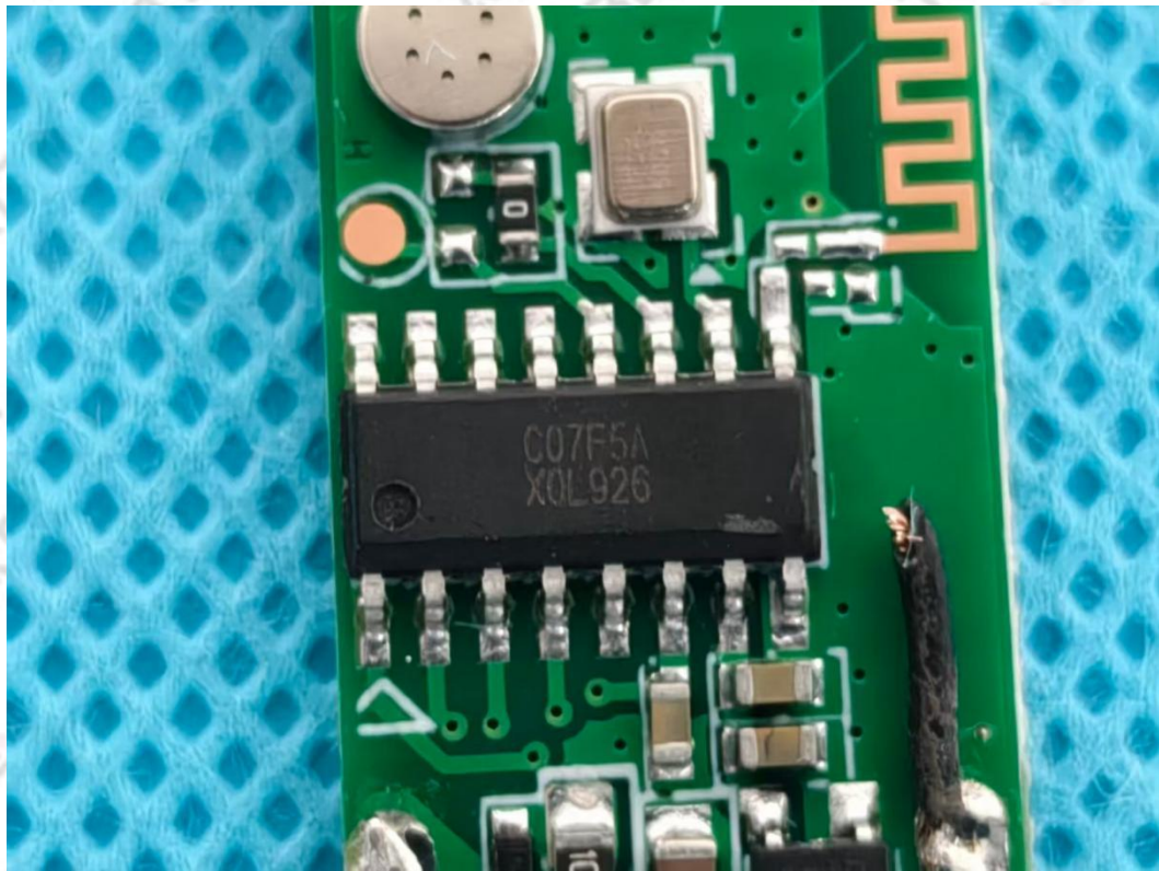
BLE_ANT
