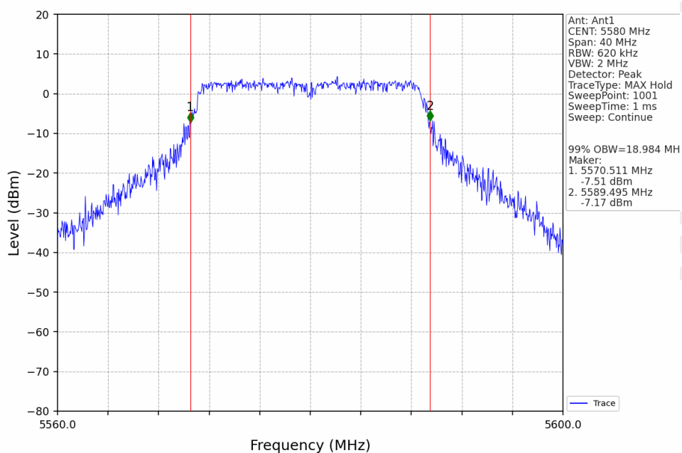
802.11n(HT20) MCH 5580MHz Ant1 NTV
