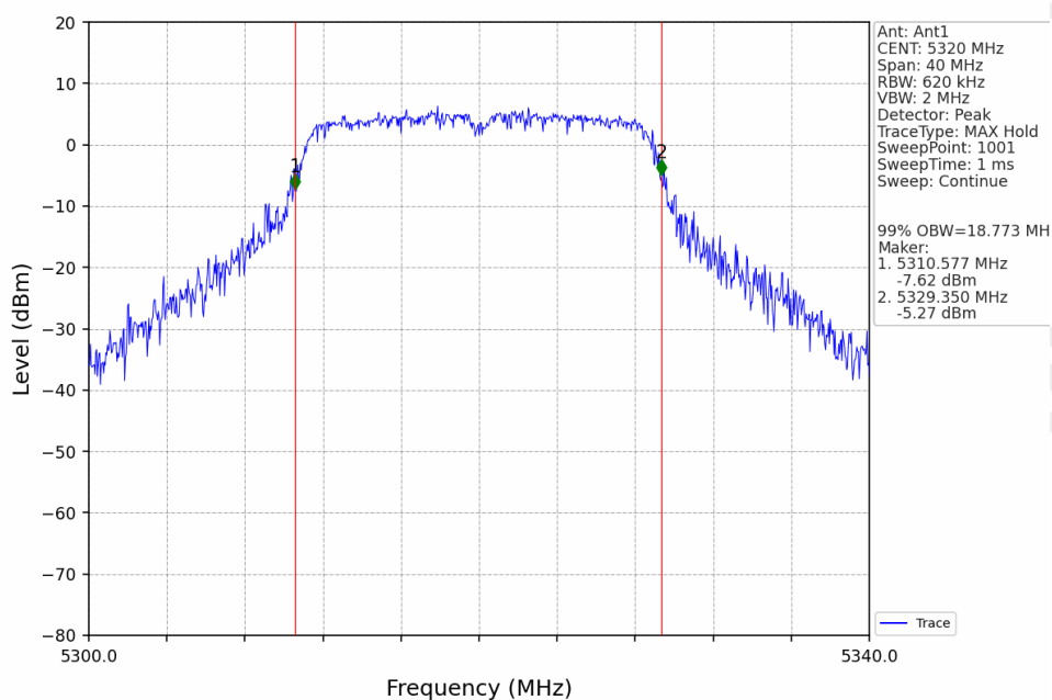
802.11n(HT20) HCH 5320MHz Ant1 NTV
