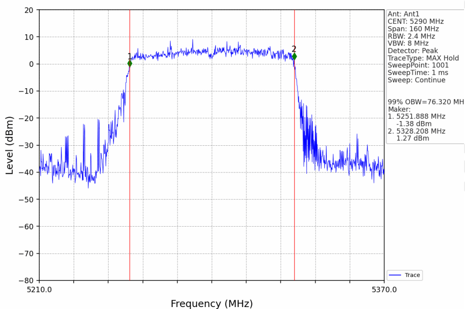
802.11ac(VHT80) MCH 5290MHz Ant1 NTVN
