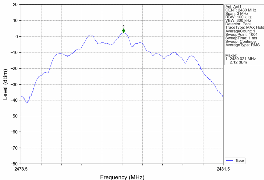
2M_HCH_2480MHz_Ant1_NTNV
