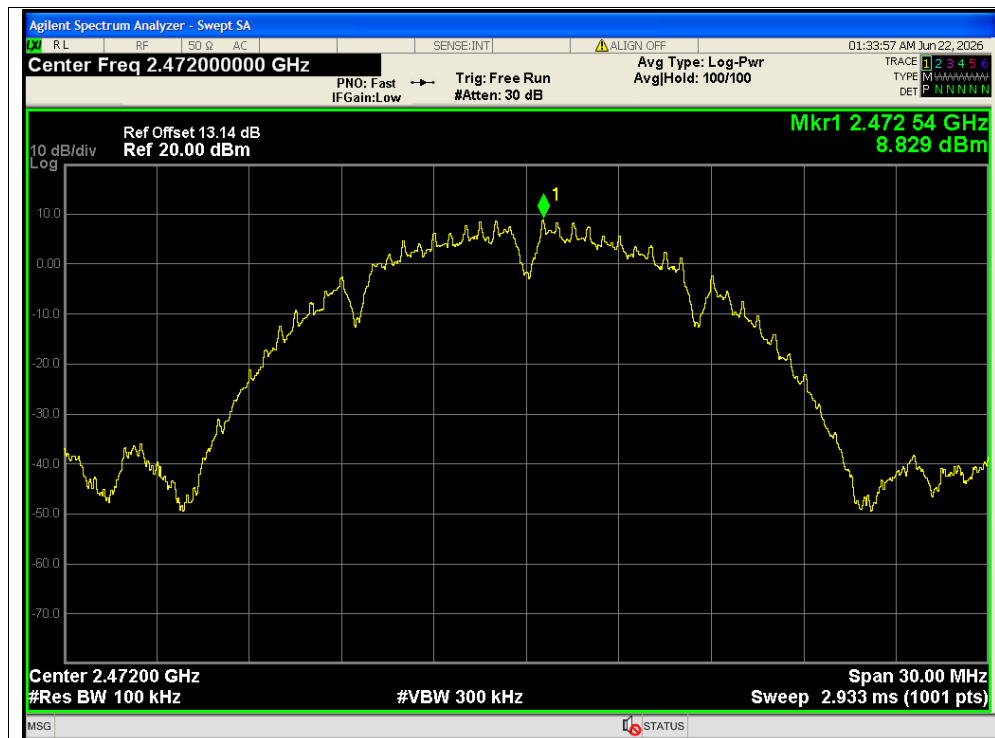
Band Edge NVNT b 2472MHz Ant1 Ref
