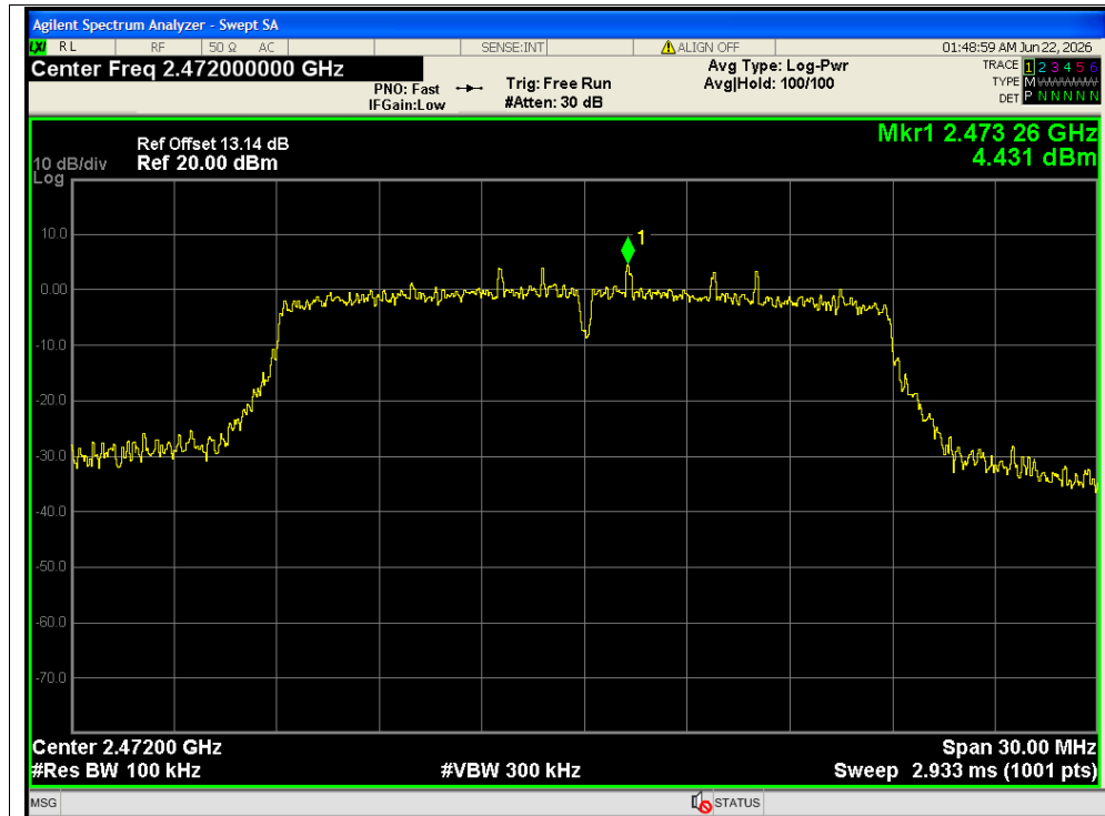
Band Edge NVNT n20 2472MHz Ant1 Ref
