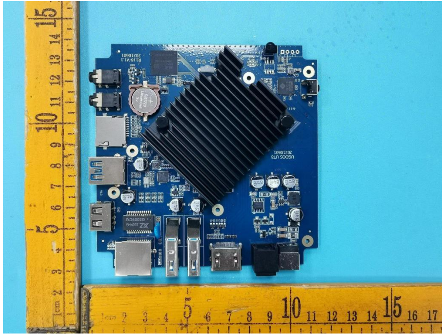
BT/2.4GWIFI/5.2G/5.8GWIFI-ANT1
