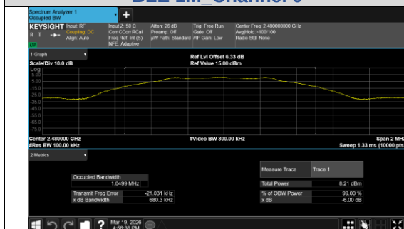
BLE 1M_Channel 39
