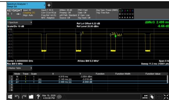
BLE 1M_Channel 19
