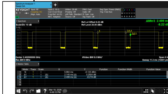
BLE 1M_Channel 0
