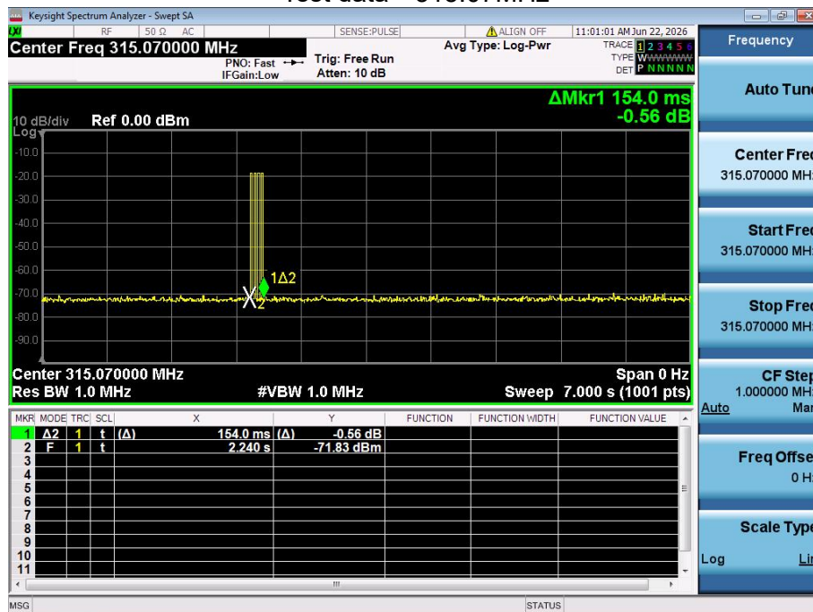
Test data—315.07MHz
