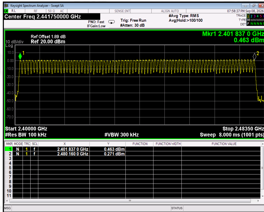
\pi/4 -DQPSK - 2-DH1 Test Plots
