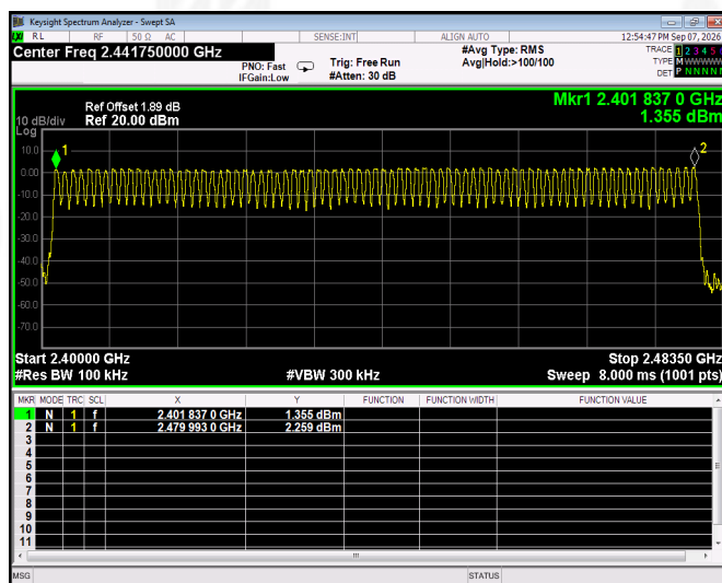
\pi/4 -DQPSK - 2-DH1 Test Plots
