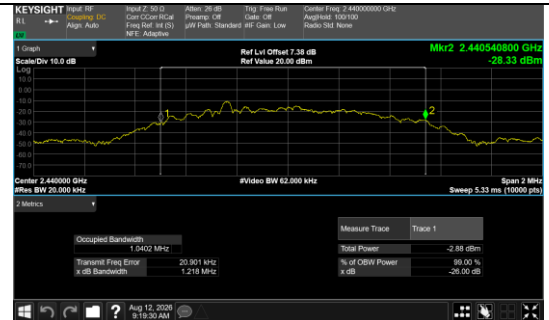
BLE 1M_Channel 19
