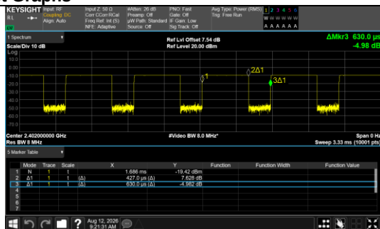
BLE 1M_Channel 0
