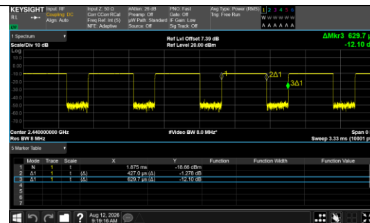
BLE 1M_Channel 19
