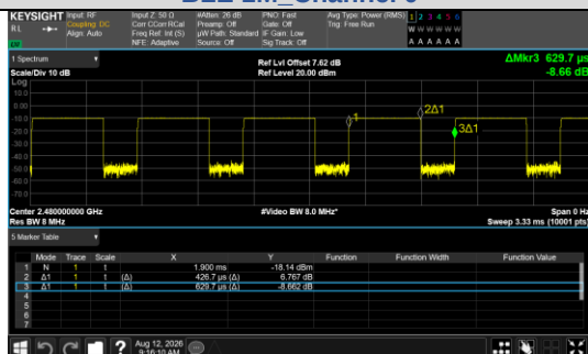
BLE 1M_Channel 39
