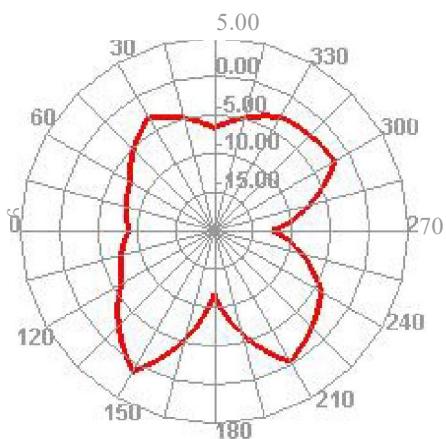
2500.000MHz
