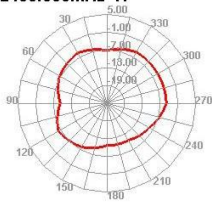
2400.000MHz E2
