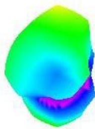
2400.000MHz
