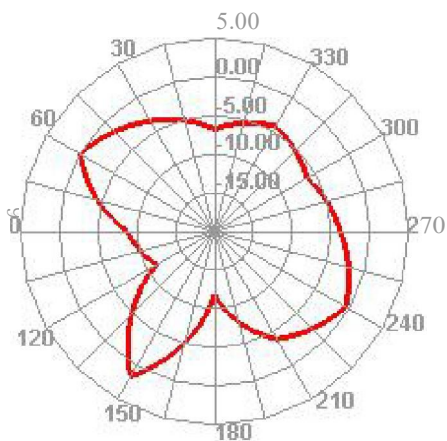
2500.000MHz H
