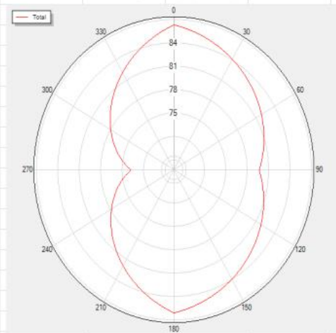
BLUETOOTH_Tis_Rssi_V78 Total
