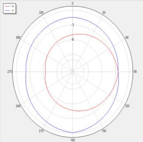
BLUETOOTH_Trp_H0 Polar
