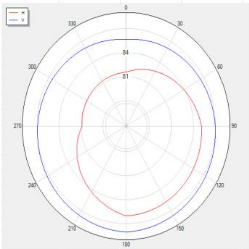
BLUETOOTH_Tis_Rssi_H39 Polar
