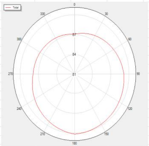
BLUETOOTH_Tis_Rssi_H39 Total
