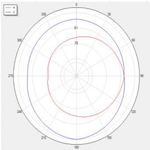
BLUETOOTH_Tis_Rssi_V0 Polar
