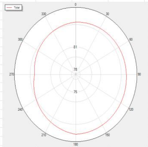
BLUETOOTH_Tis_Rssi_V0 Total
