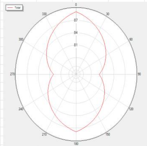
BLUETOOTH_Tis_Rssi_V39 Total
