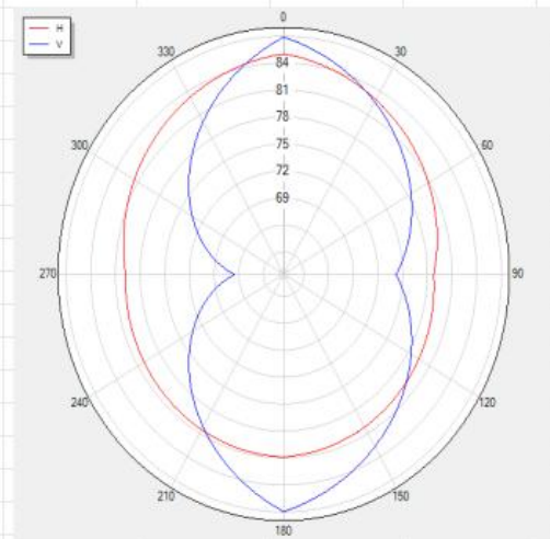
BLUETOOTH_Tis_Rssi_V39 Polar
