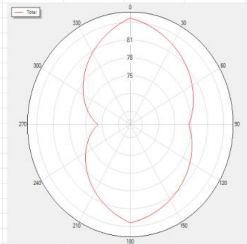
BLUETOOTH_Tis_Rssi_V0 Total
