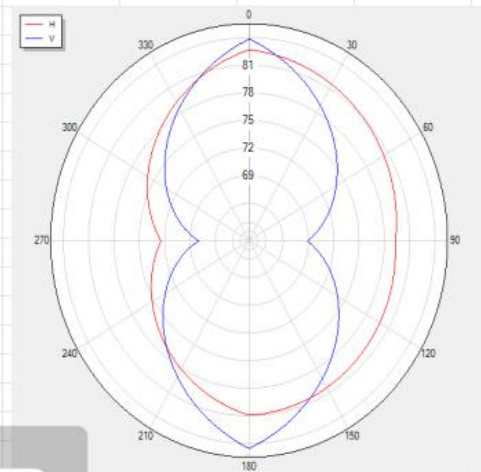
BLUETOOTH_Tis_Rssi_V78 Polar
