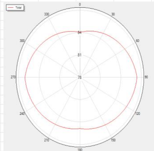
BLUETOOTH_Tis_Rssi_H78 Total
