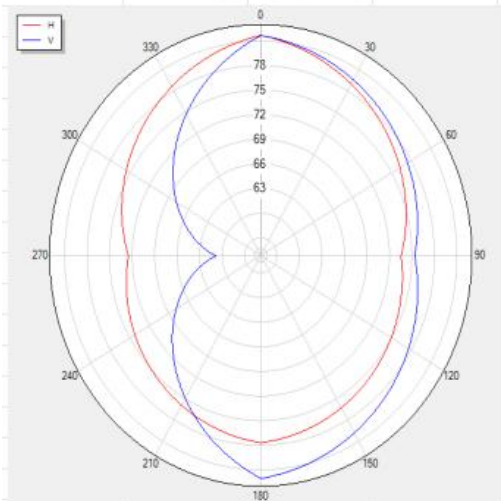
BLUETOOTH_Tis_Rssi_V0 Polar
