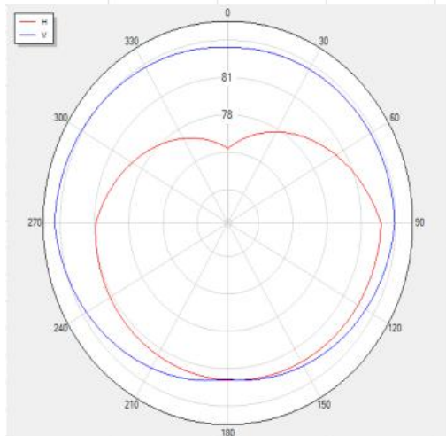
BLUETOOTH_Tis_Rssi_H78 Polar
