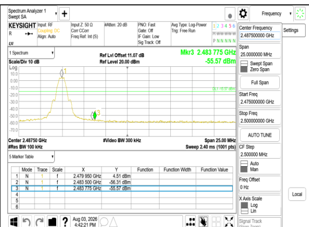
Band Edge BLE 1M 2480MHz
