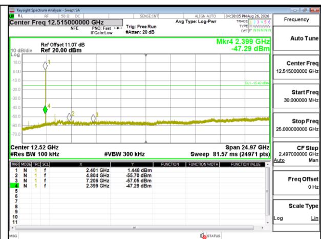
Spurious Emission BLE 2M 2402MHz
