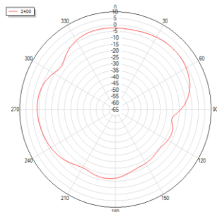
Theta=90 freq=2400MHz
