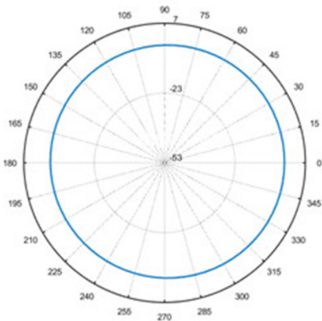
Total-Polar-H-690MHZ
