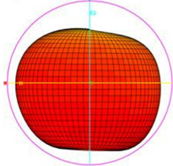
Total-3D-E1-665MHZ
