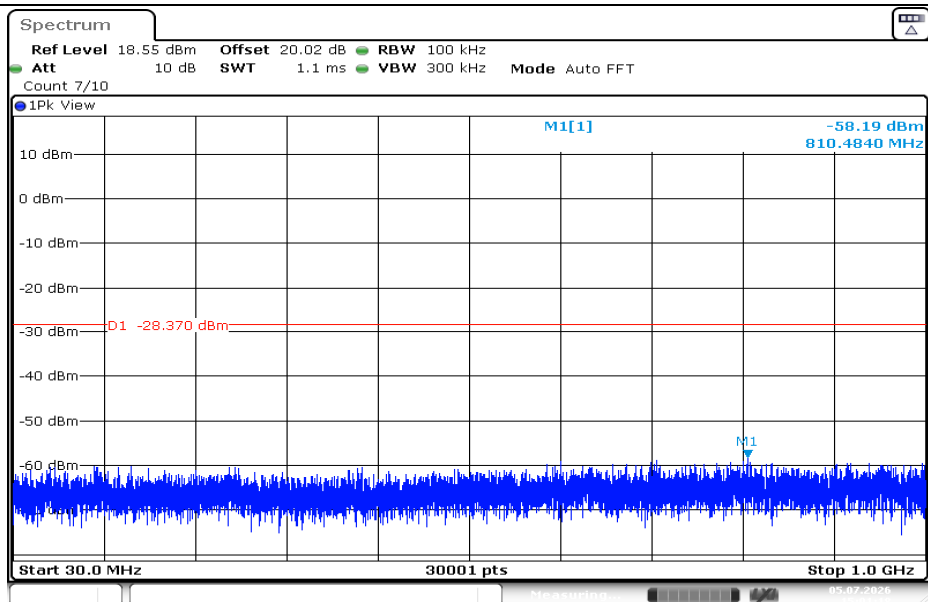
11G-Ant1-2462-30~1000-PASS
