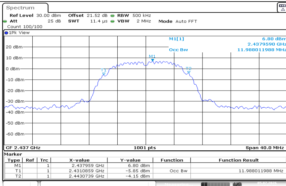
11B-Ant1-2437
