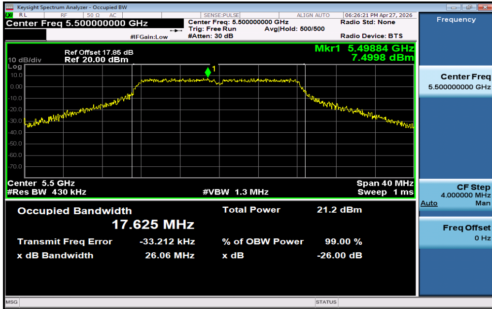
11A-Ant1-5500
