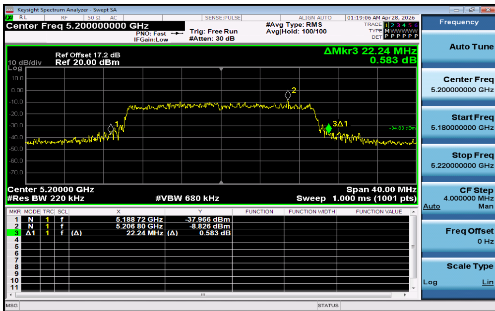
11AX20SISO-Ant1-5200
