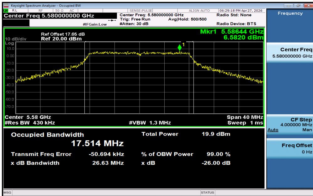
11A-Ant1-5580
