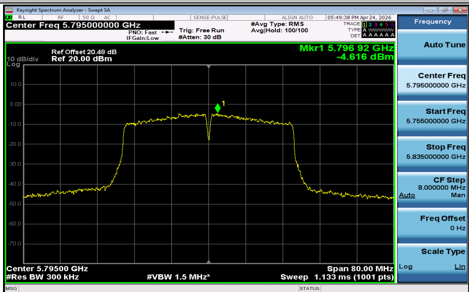
11AX40SISO_Ant1_5795
