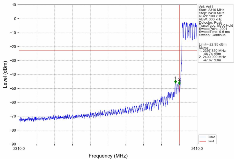
2.4G_HOPP_Ant1_NTNV
