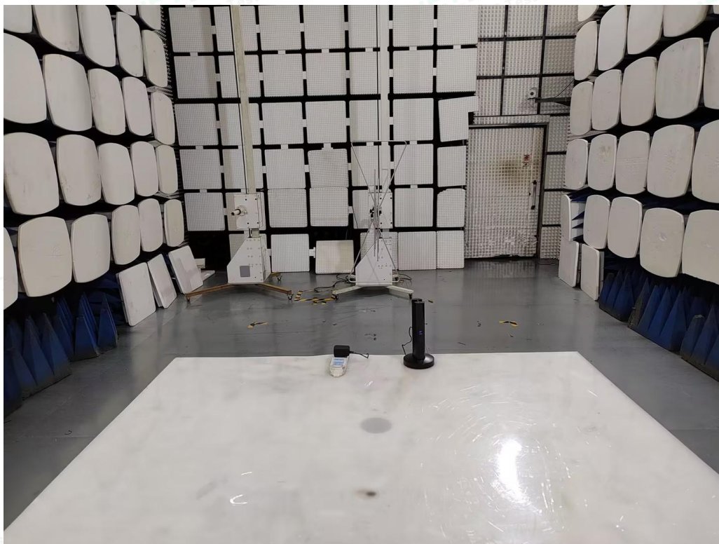
Fig. 1 (30MHz~1GHz)
