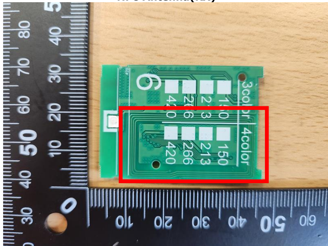
NFC Antenna(RX)
