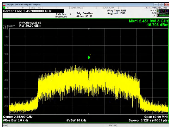
802.11ax40 - CH09
