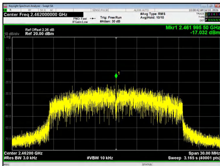
802.11ax20 - CH11
