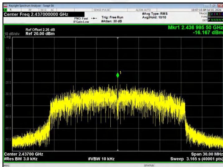
802.11ax20 - CH06
