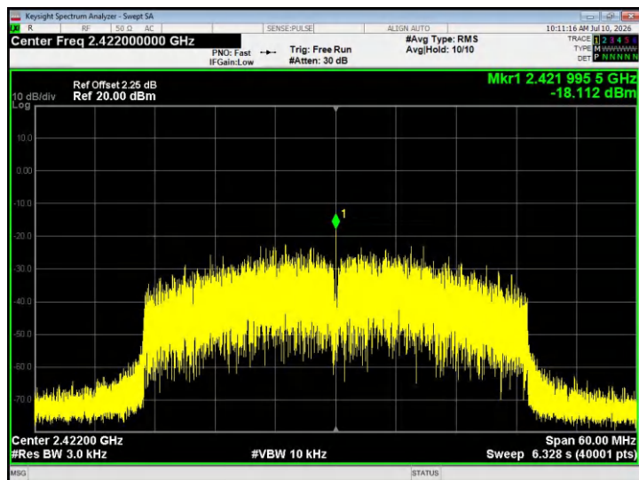
802.11ax40 - CH03
