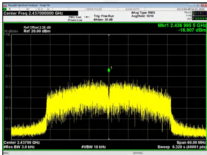
802.11ax40 - CH06
