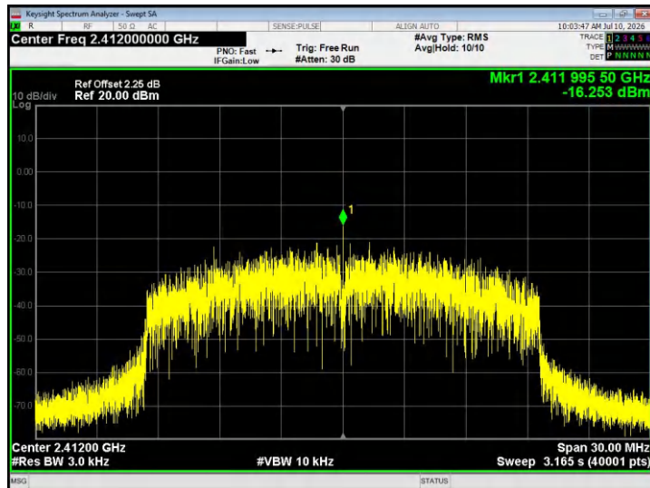
802.11ax20 - CH01
