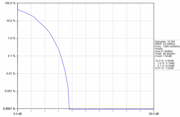
Band2_20MHz_16QAM_MCH_1880MHz_RB_27_0_NTNV
