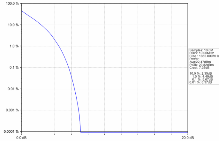
Band2_10MHz_QPSK_LCH_1855MHz_RB_50_0_NTNV
