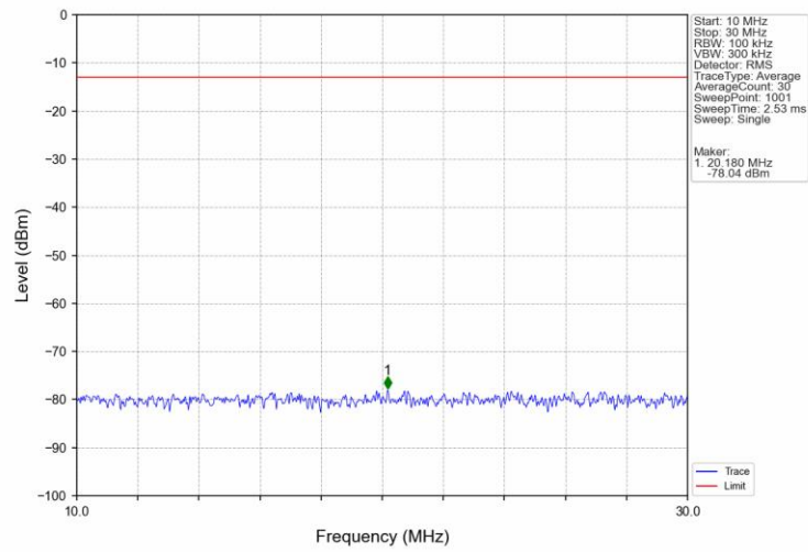
Band2_1.4MHz_QPSK_HCH_1909.3MHz_RB_1_0_NTNV
