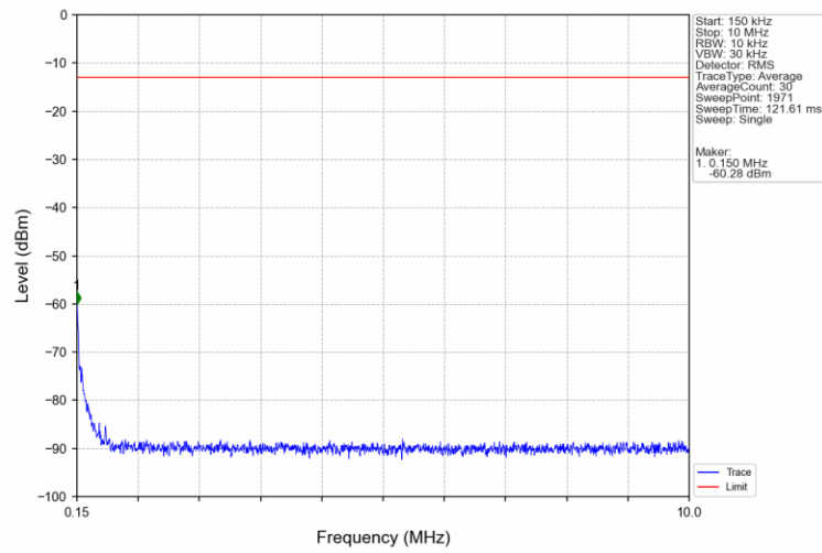
Band2_1.4MHz_QPSK_MCH_1880MHz_RB_1_0_NTNV
