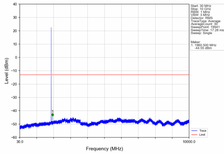
Band2_1.4MHz_QPSK_MCH_1880MHz_RB_1_0_NTNV
