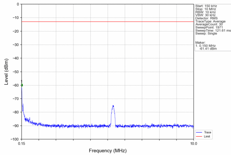
Band4_20MHz_QPSK_LCH_1720MHz_RB_1_0_NTNV
