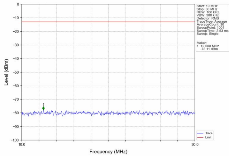
Band4_20MHz_QPSK_HCH_1745MHz_RB_1_0_NTNV
