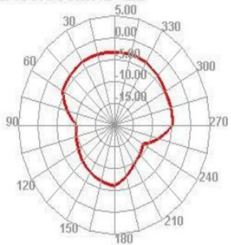
2480.000MHz E2
