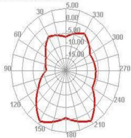
2450.000MHz H
