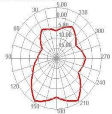
2500.000MHz H
