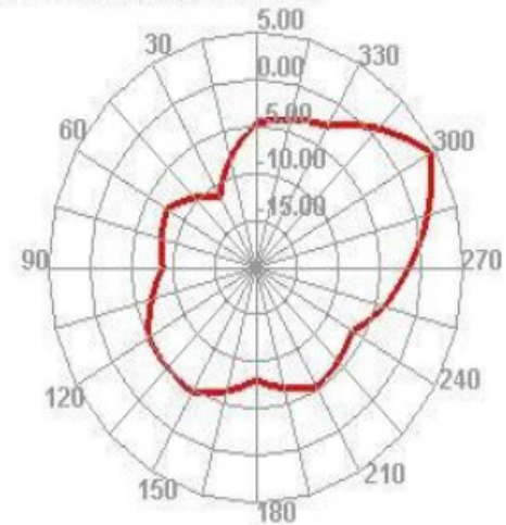
2400.000MHz E1
