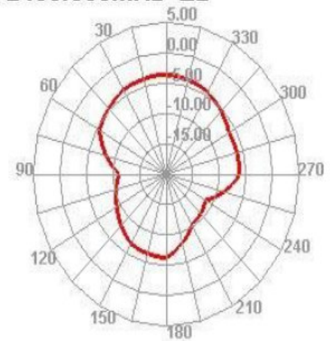
2450.000MHz E2
