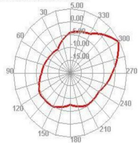
2420.000MHz E1
