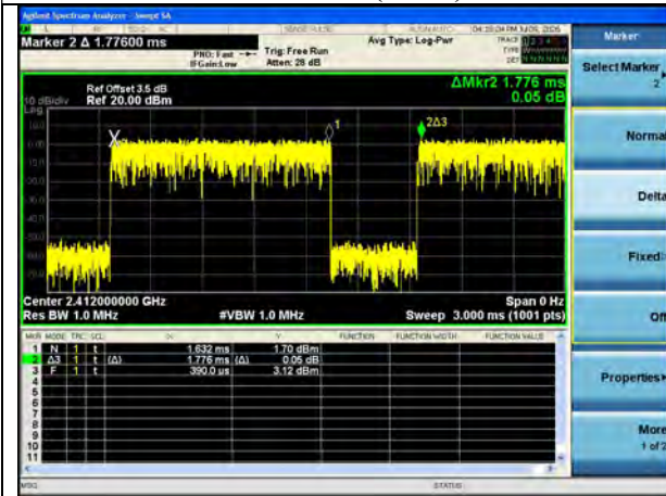
802.11n20(MHz)
