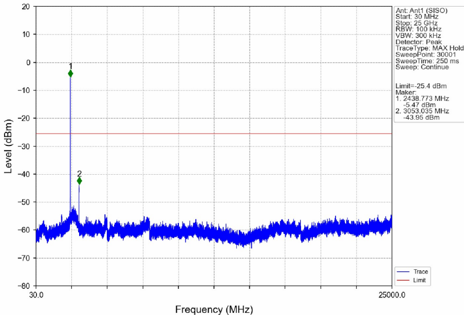
802.11g_MCH_2437MHz_Ant1 (SISO)_NTNV
