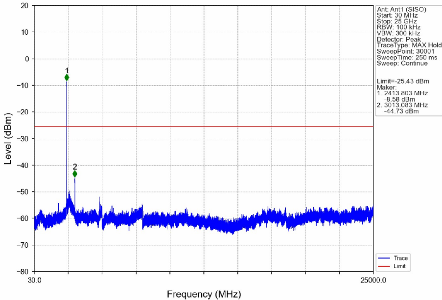
802.11g_MCH_2437MHz_Ant1 (SISO)_NTNV
