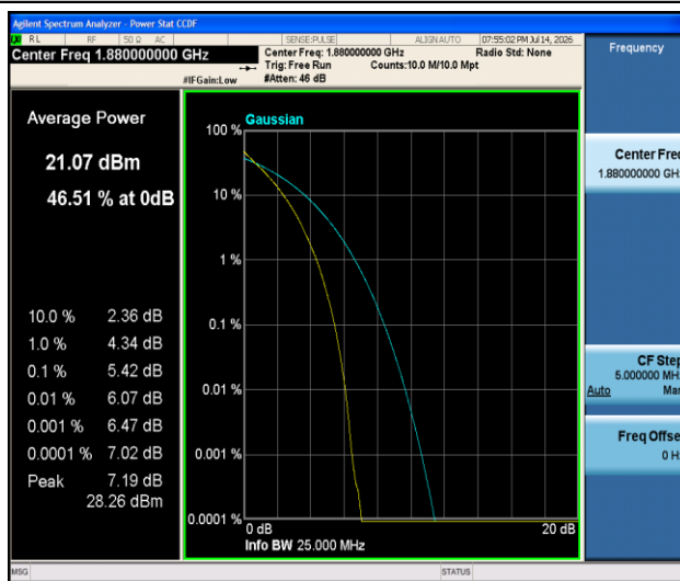
Band2-20MHz-QPSK-18900-100RB#0-PASS
