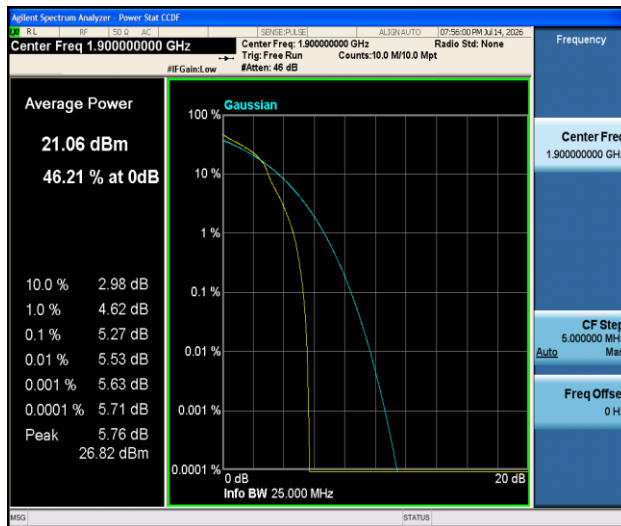
Band2-20MHz-16QAM-19100-1RB#0-PASS
