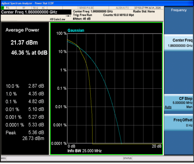
Band2-20MHz-16QAM-18700-1RB#0-PASS
