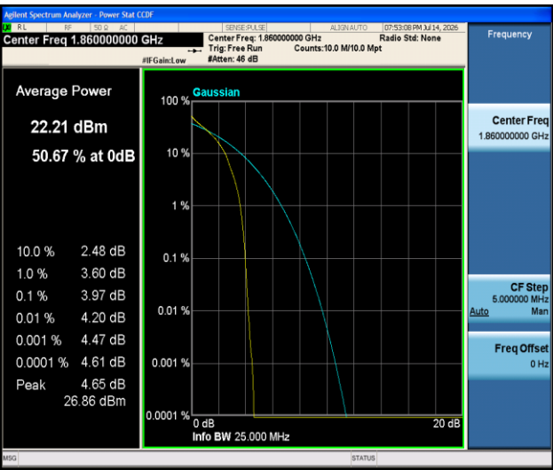
Band2-20MHz-QPSK-18700-1RB#0-PASS
