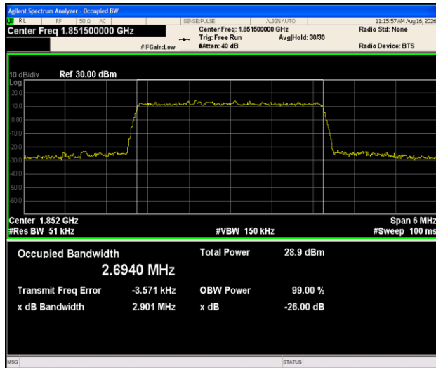
Band2-3MHz-QPSK-18615-15RB#0-PASS
