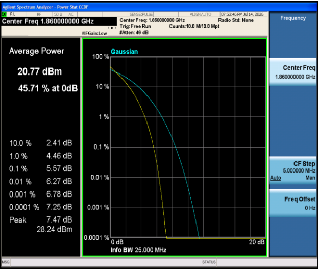
Band2-20MHz-QPSK-18700-100RB#0-PASS
