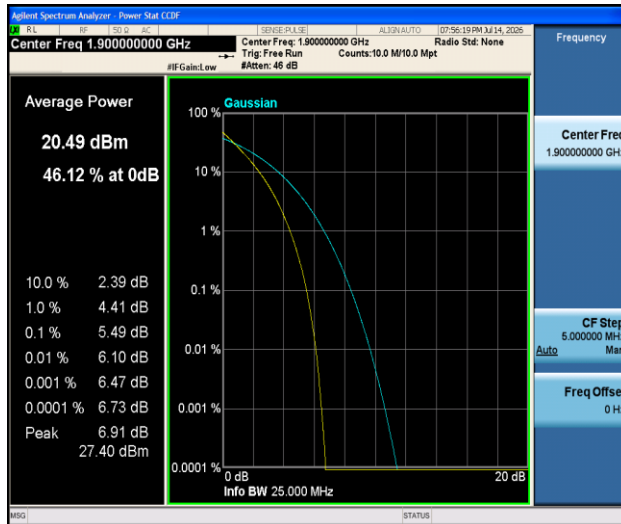
Band2-20MHz-QPSK-19100-100RB#0-PASS
