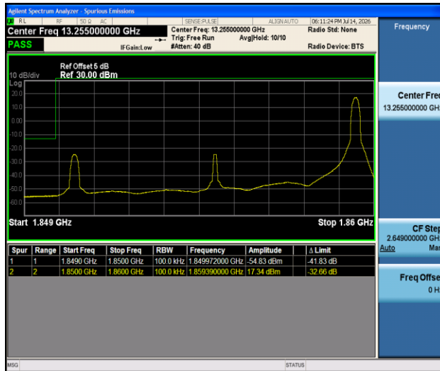
Band2-10MHz-QPSK-18650-1RB#49-PASS
