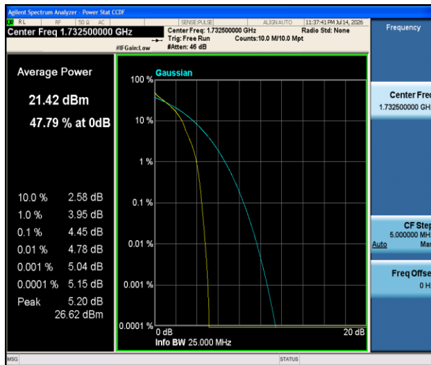
Band4-20MHz-QPSK-20175-1RB#0-PASS
