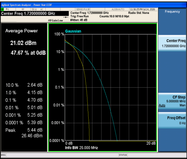
Band4-20MHz-QPSK-20050-1RB#0-PASS
